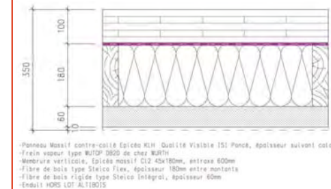
M2 / Complexe MUR Enduit
