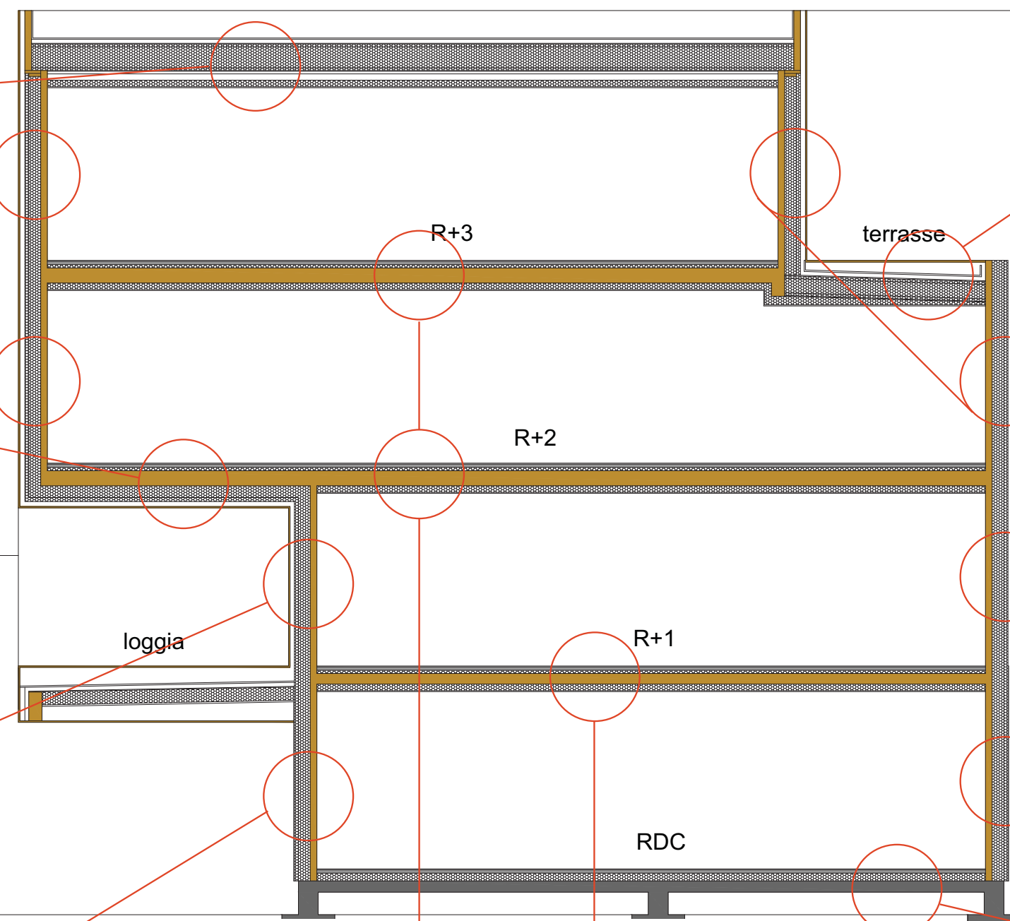
Pi1 / Complexe PLANCHER CLT 230
