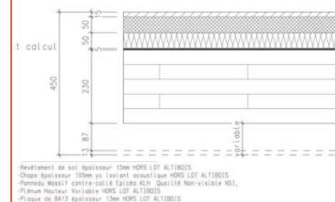
Pi1 / Complexe PLANCHER CLT 230
