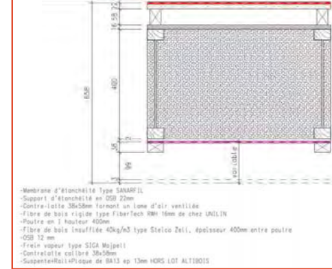
Pi1 / Complexe PLANCHER Isolé
