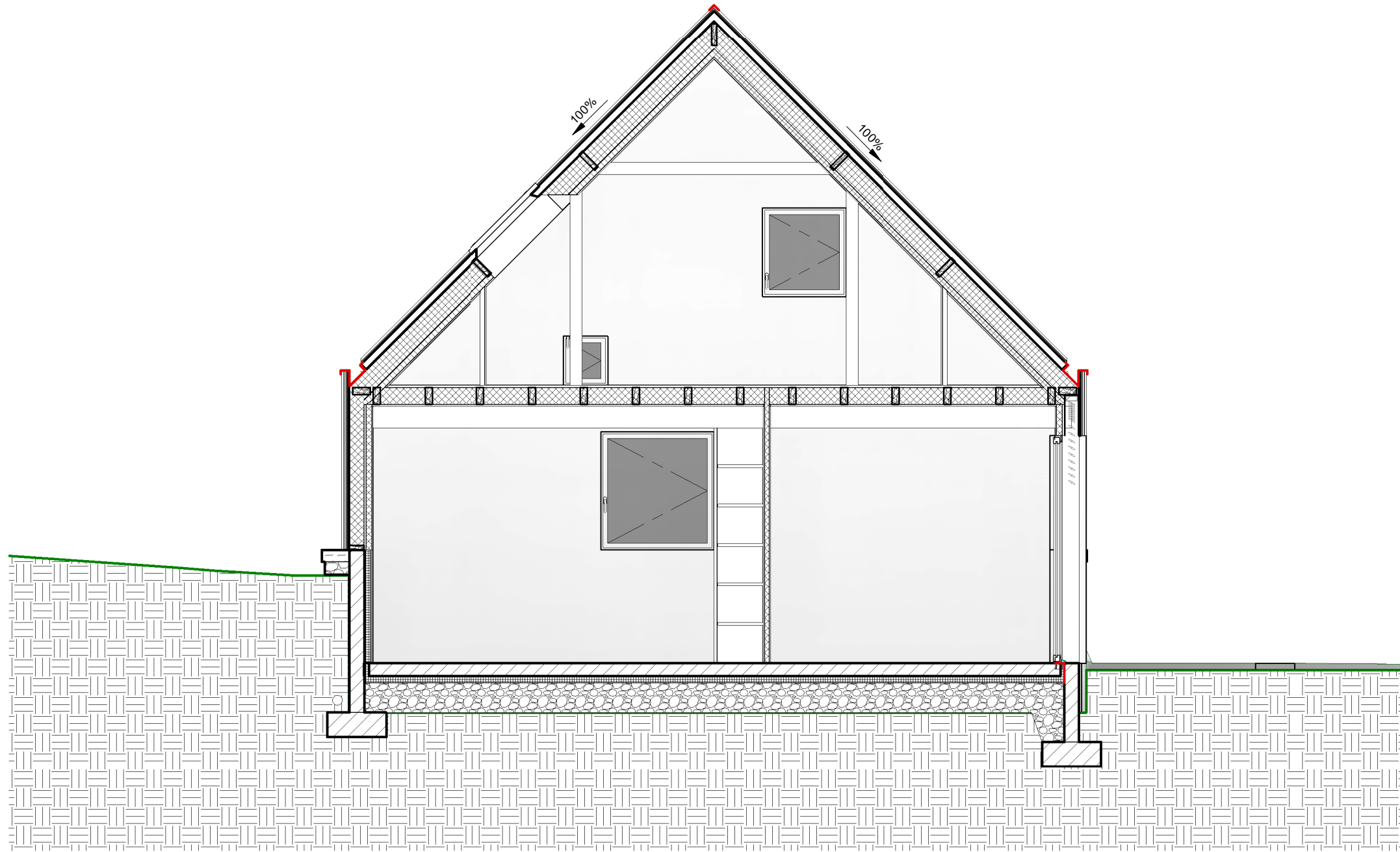
Coupe 1 : 50
