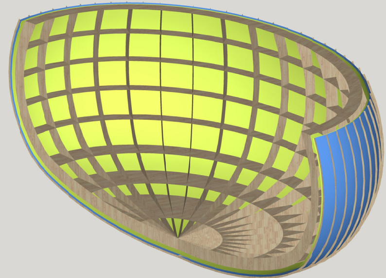
④ OSSATURE SECONDAIRE POUR LA FINITION EXTERIEURE
