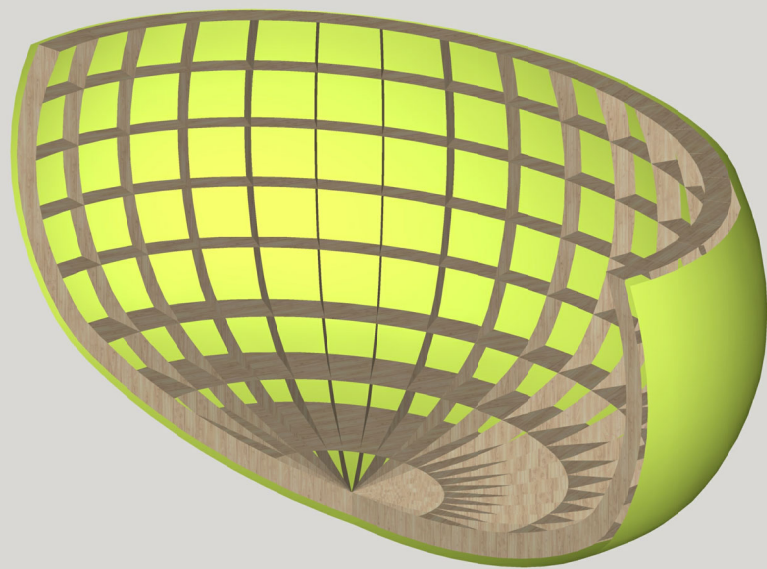
② DOUBLE-PEAU CONTRE-PLAQUÉ FINITION BOULEAU VERNIS NEUTRE SATINÉ
