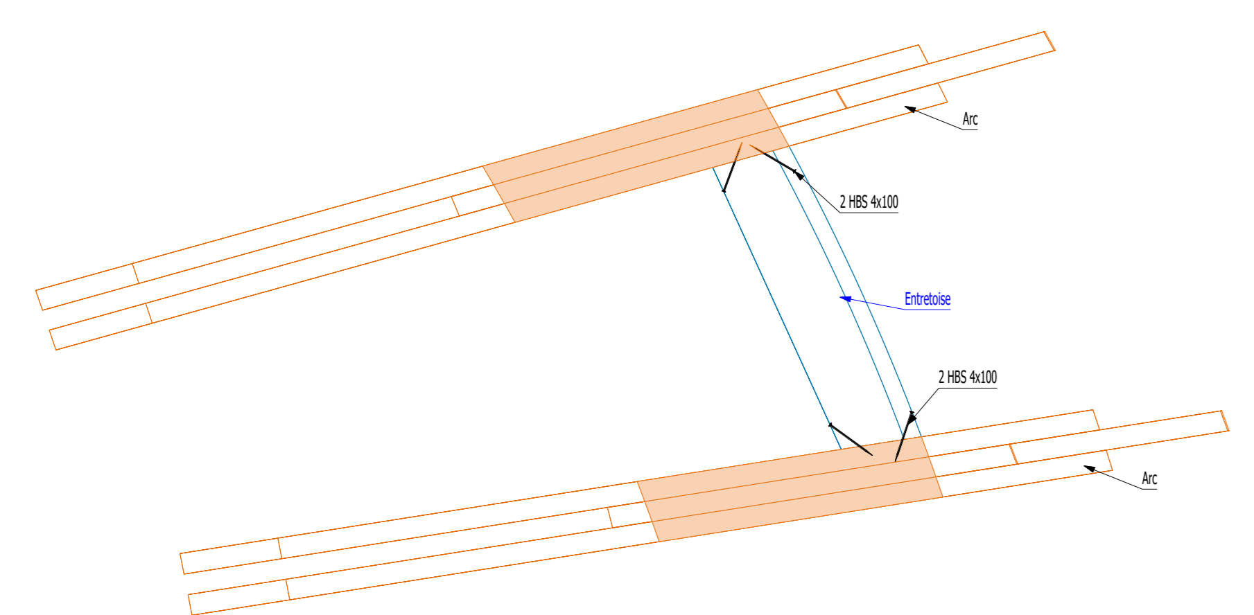
DETAIL FIXATION ENTRETOISE Ech: 1/10
