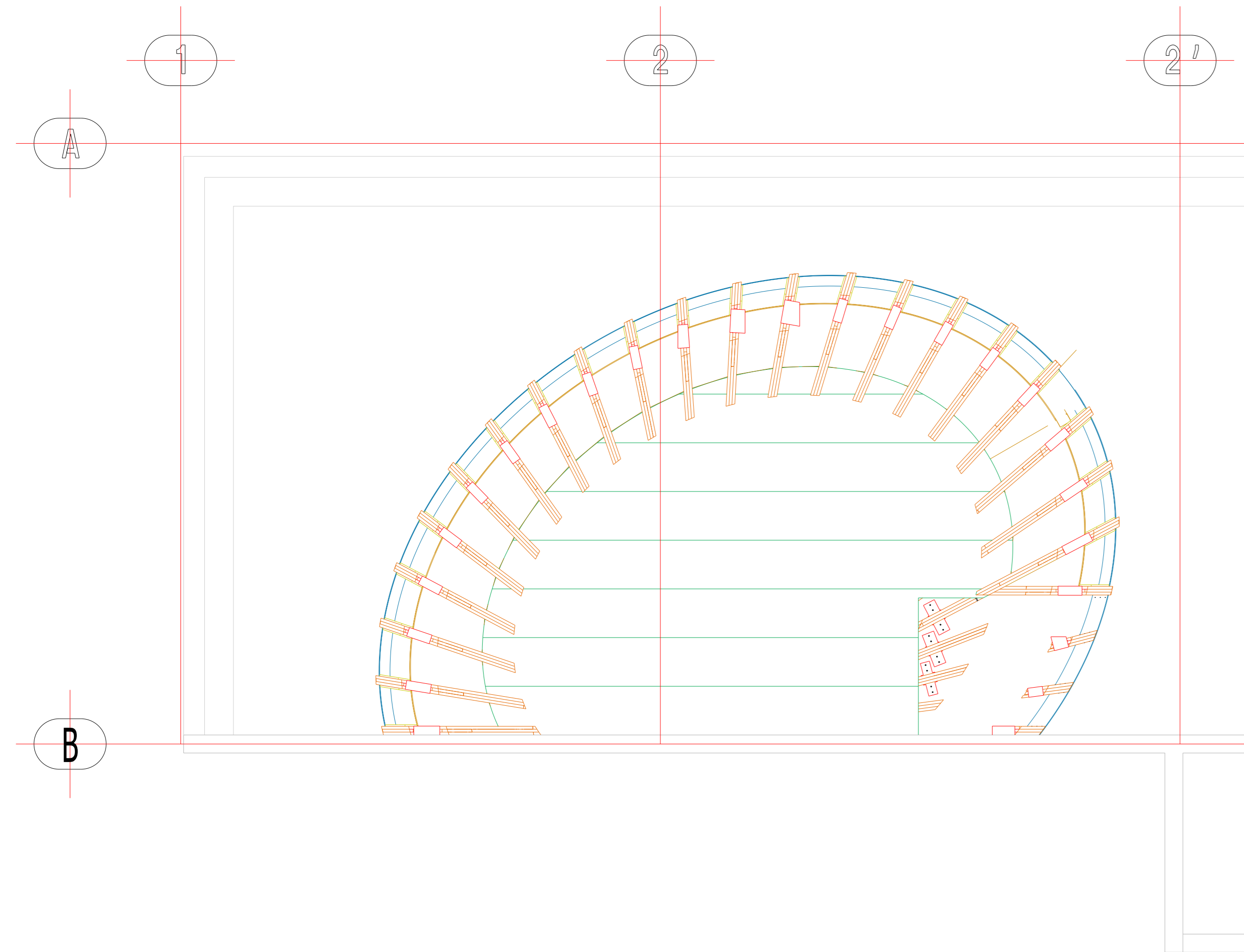
Ech: 1/25 e VUE EN PLAN OSB
