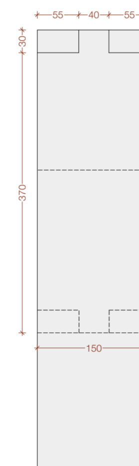
DÉTAIL 3 échelle 1/5ème
