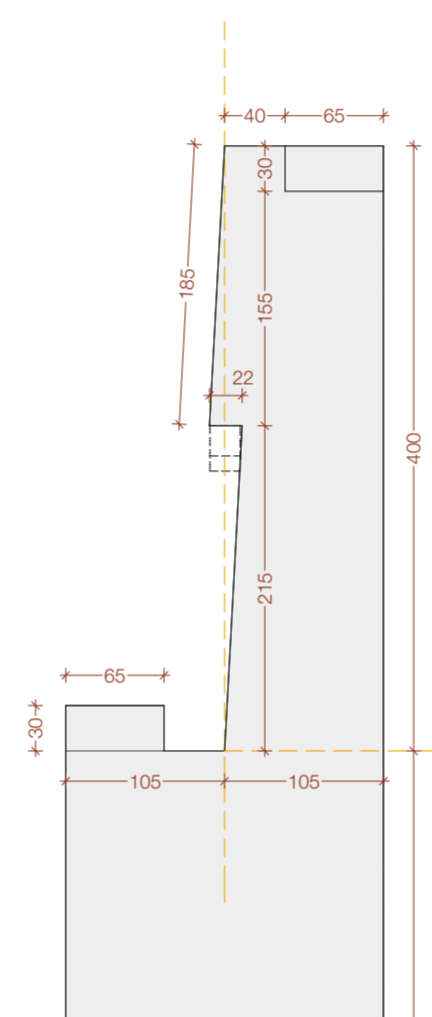
DÉTAIL 2 échelle 1/5ème
