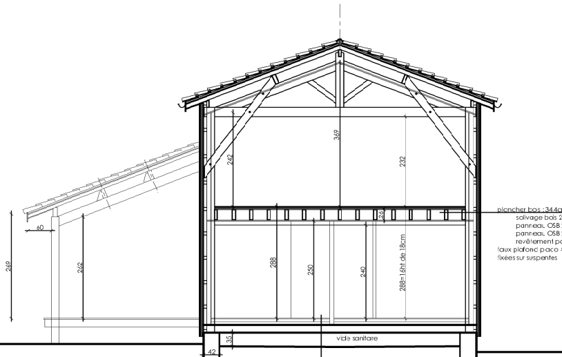
COUPE DE PRINCIPE COIN NUIT
