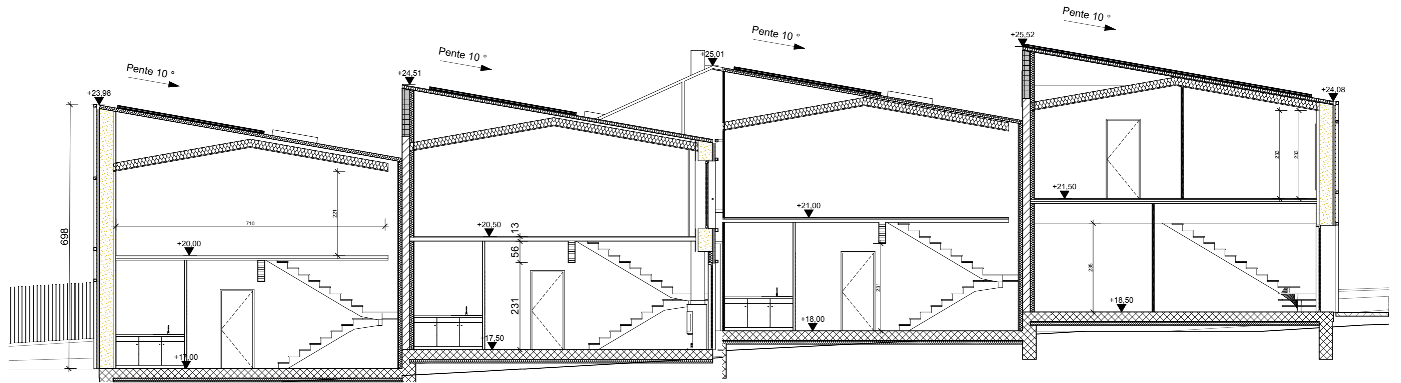
Coupe BB
