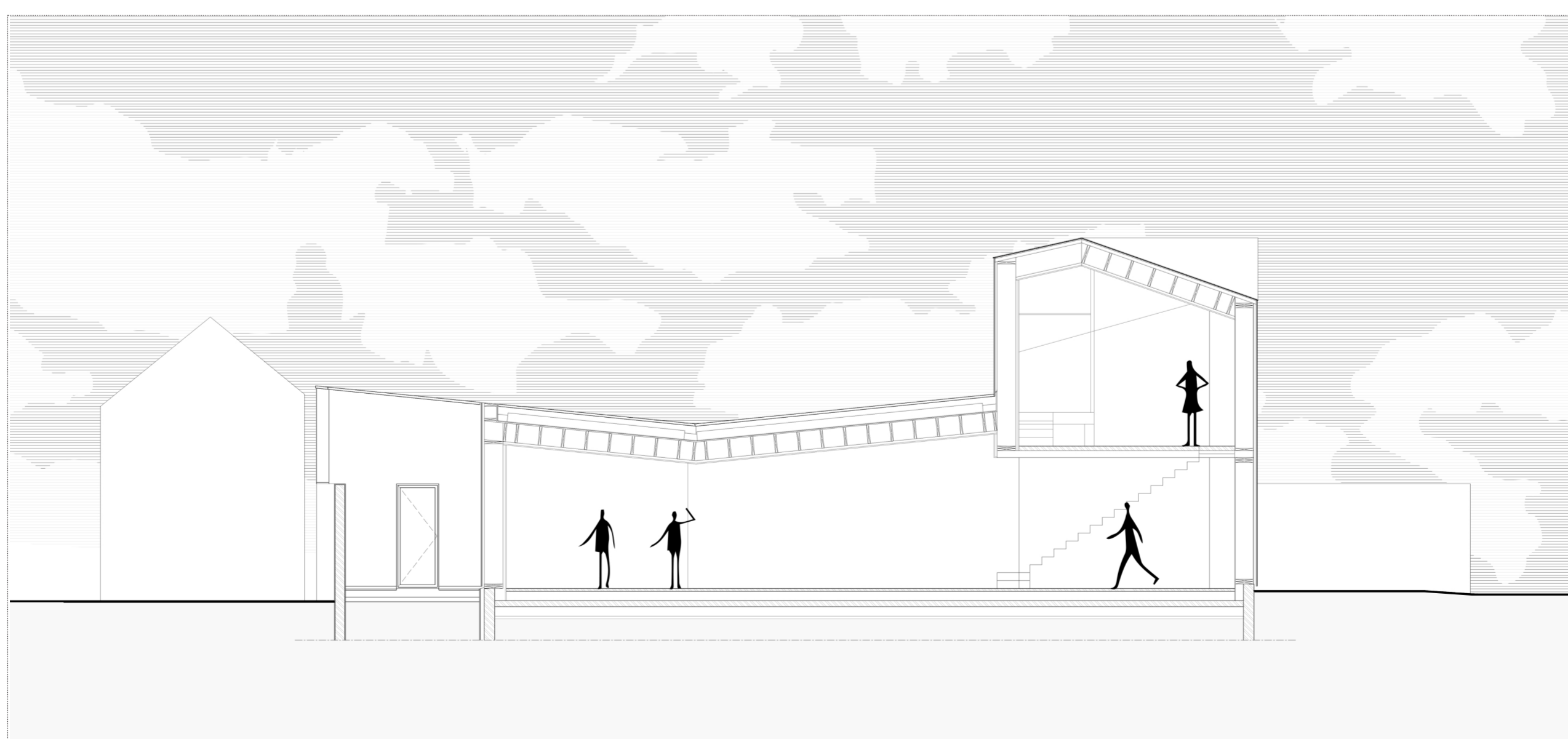
COUPE AA' échelle 1/100
