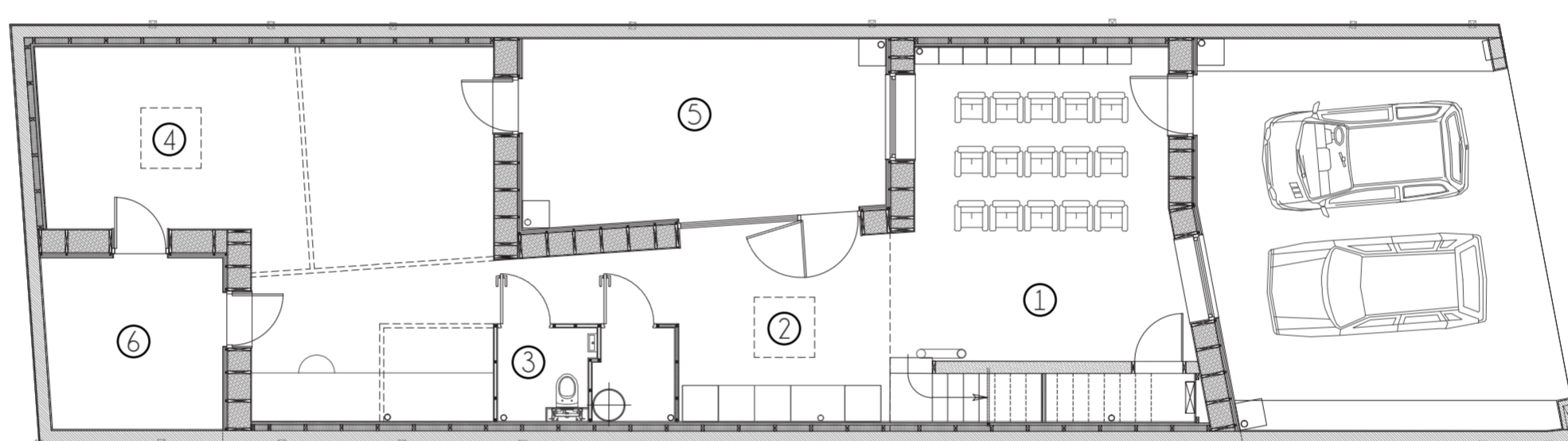
PLAN DU RDC | ⊖ échelle 1/100
