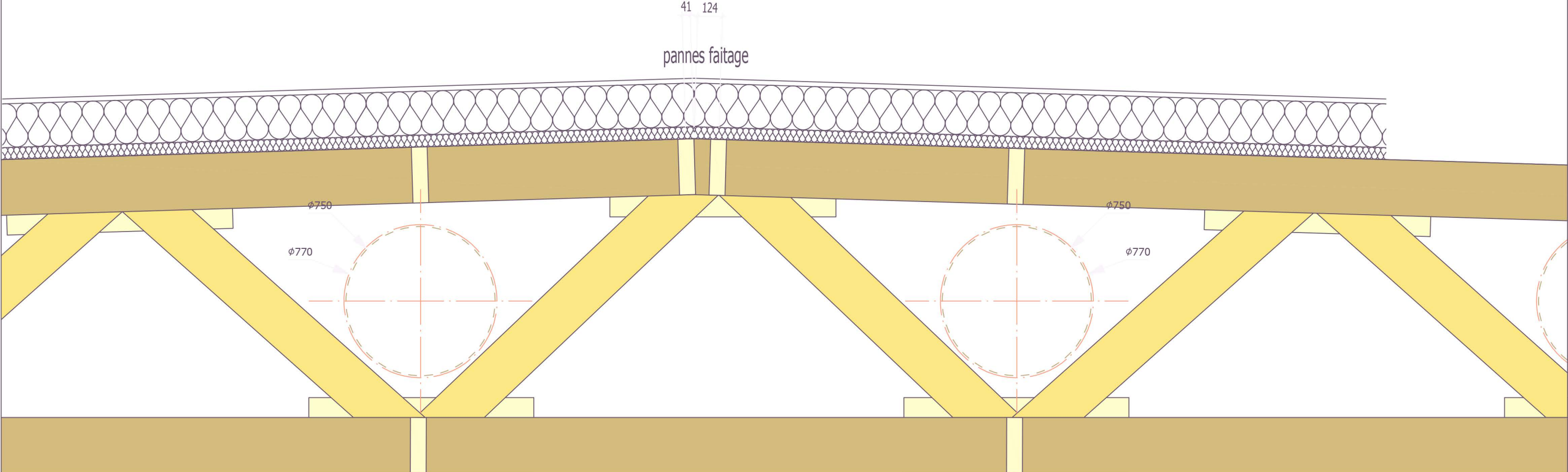
Ferme Secondaire (Poutre treillis à Inertie Variable)
