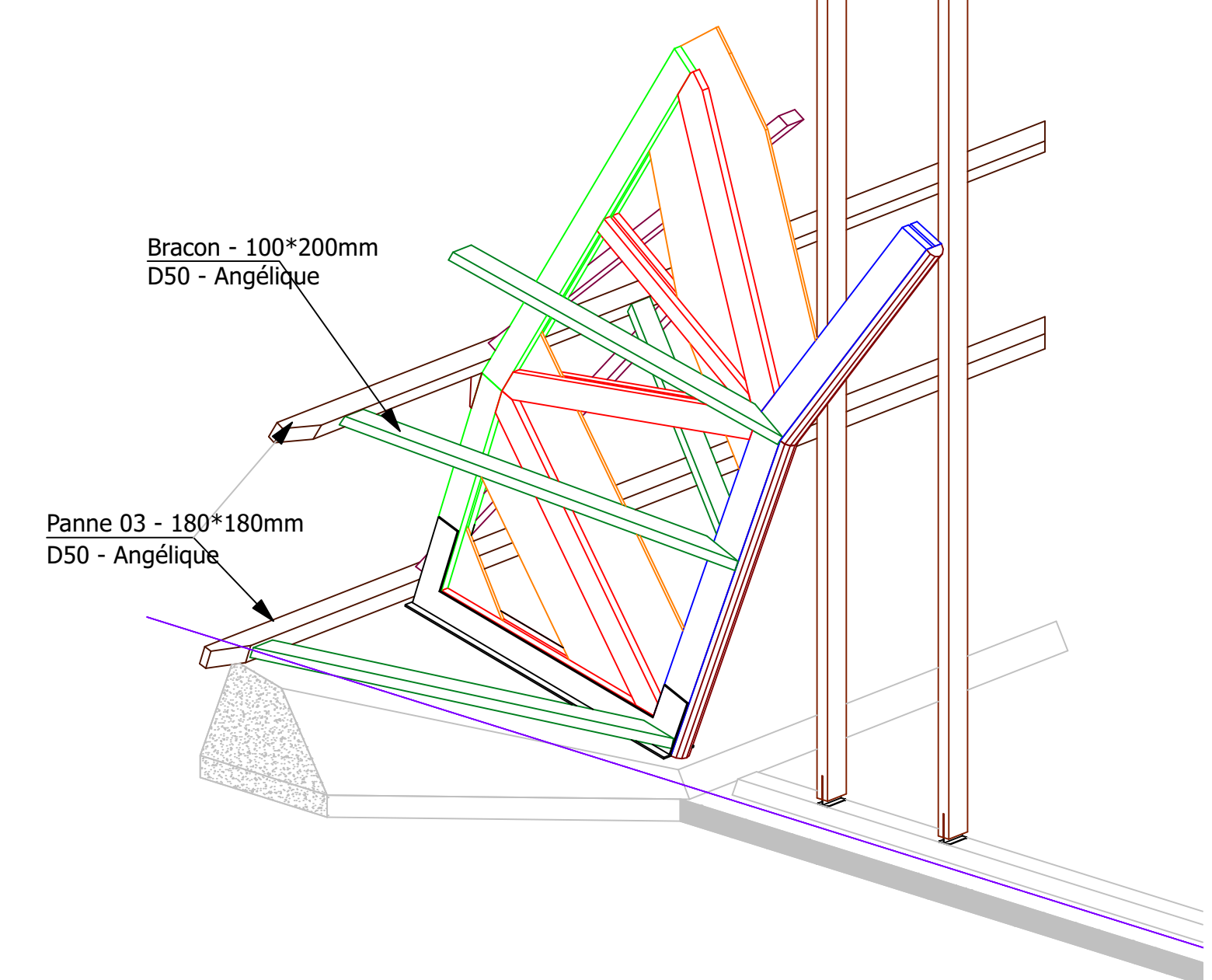
Détail 5 ASSEMBLAGE PIED DE PORTIQUE ECH:1/25
