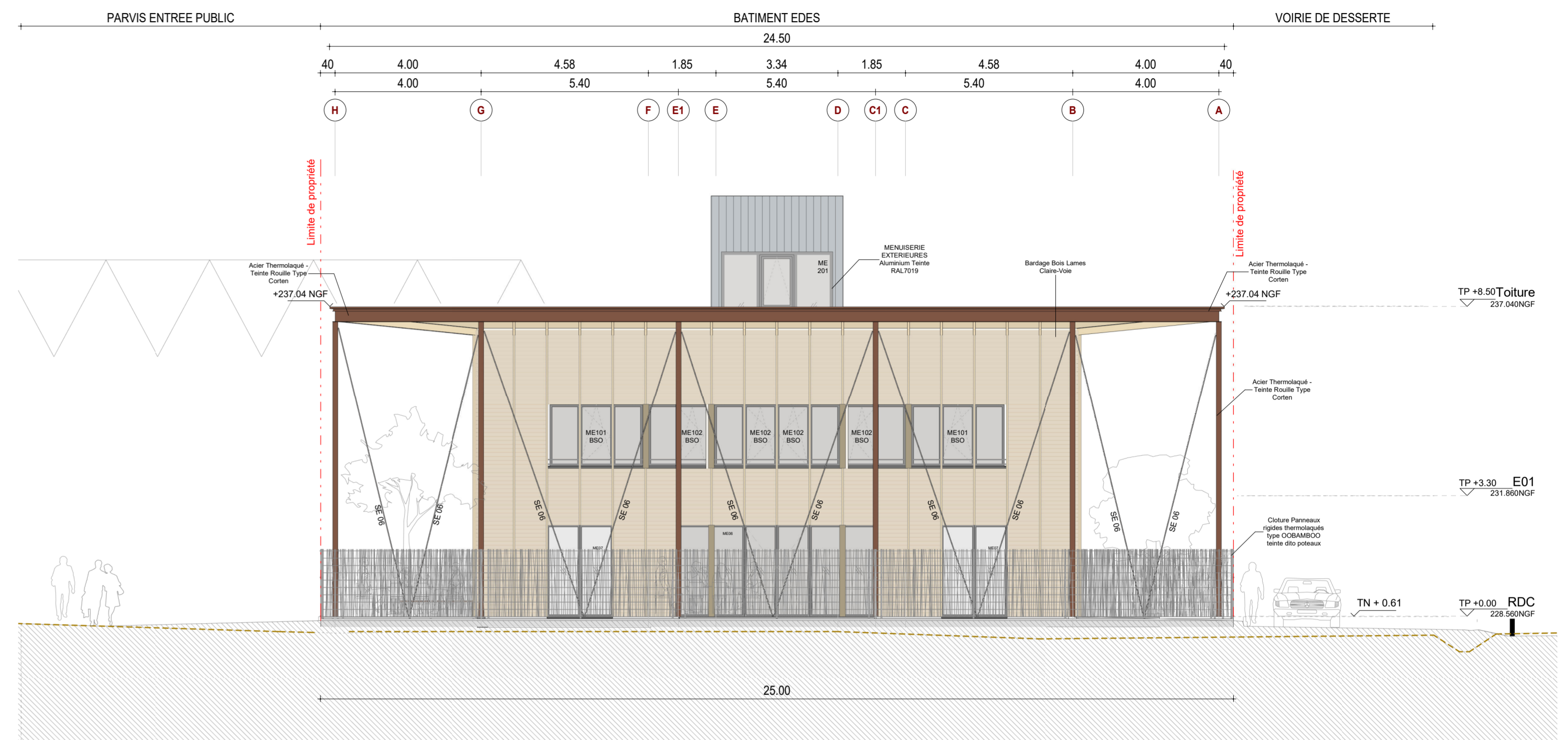
Élévation Sud-Est 1 : 100
