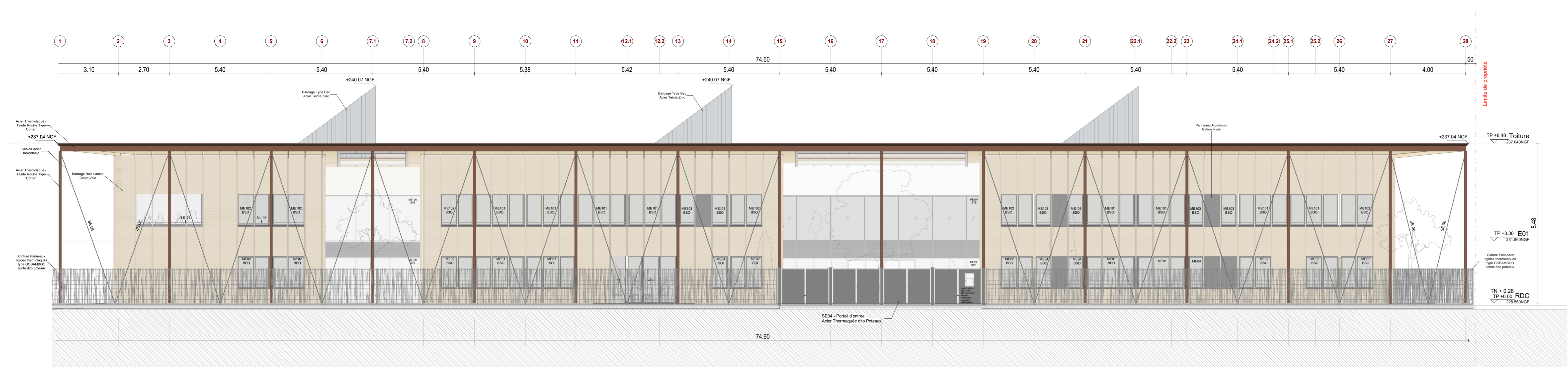
Élévation Sud-Ouest 1 : 100
