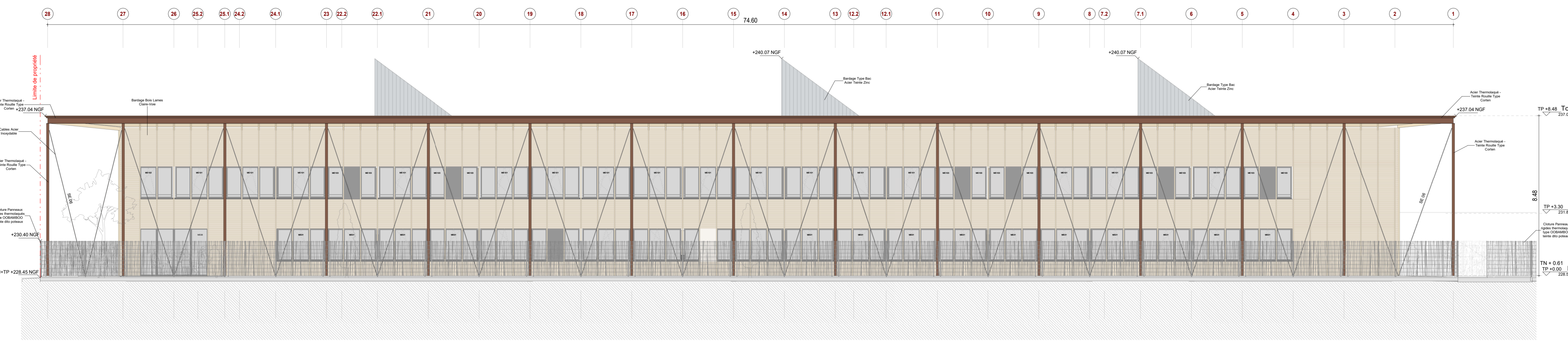
Élévation Nord-Est 1 : 100
