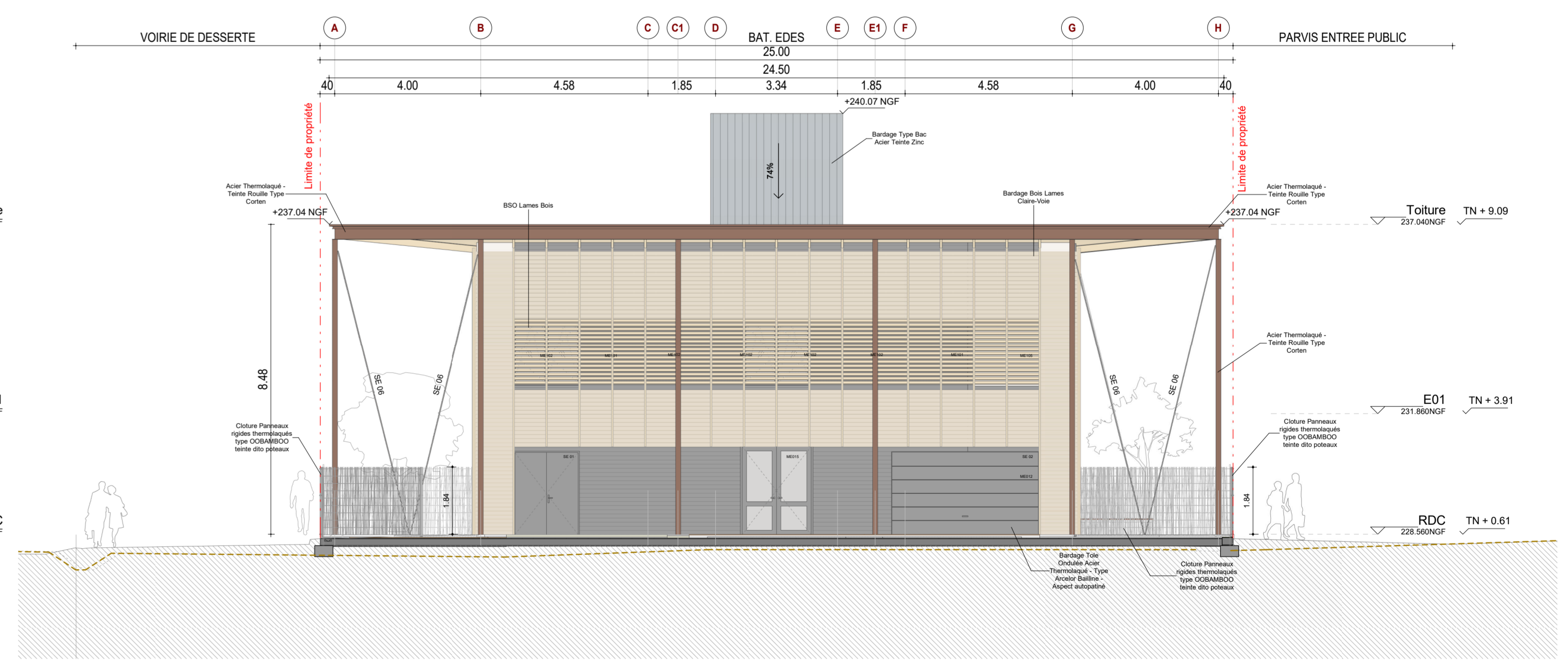
Élévation Nord-Ouest 1 : 100
