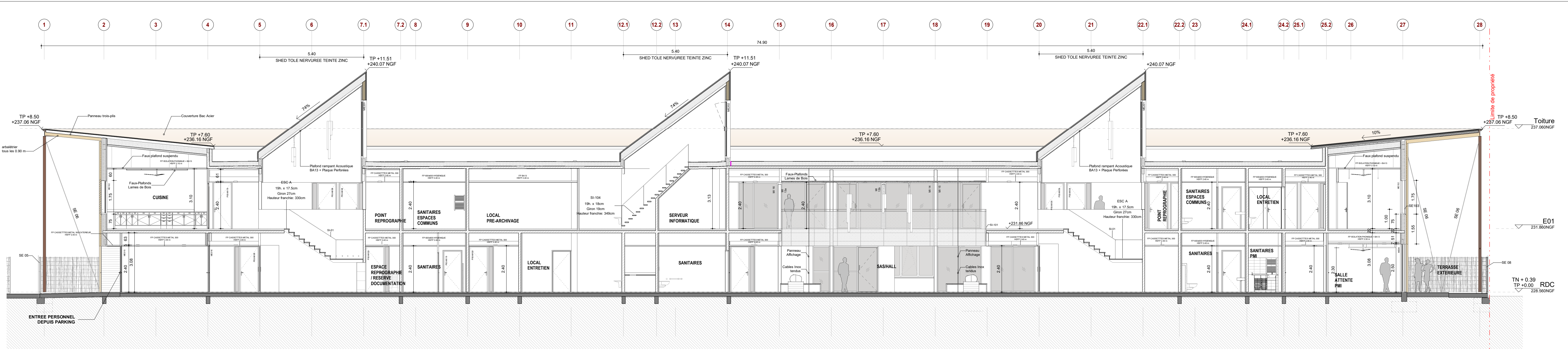
Coupe longitudinale DD' 1 : 100
