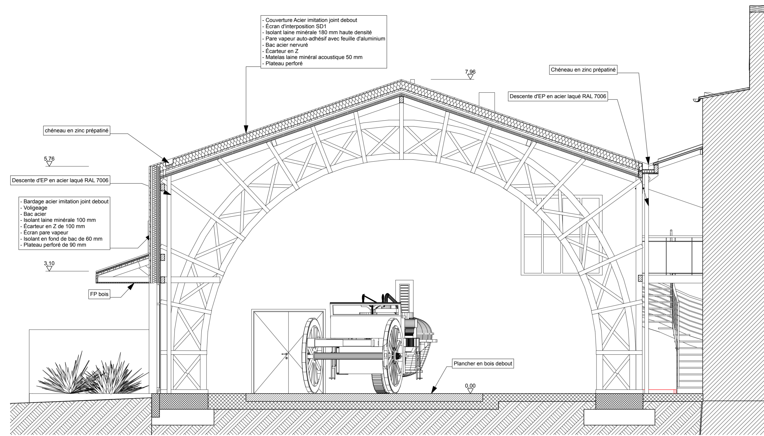
C Coupe C 1:50
