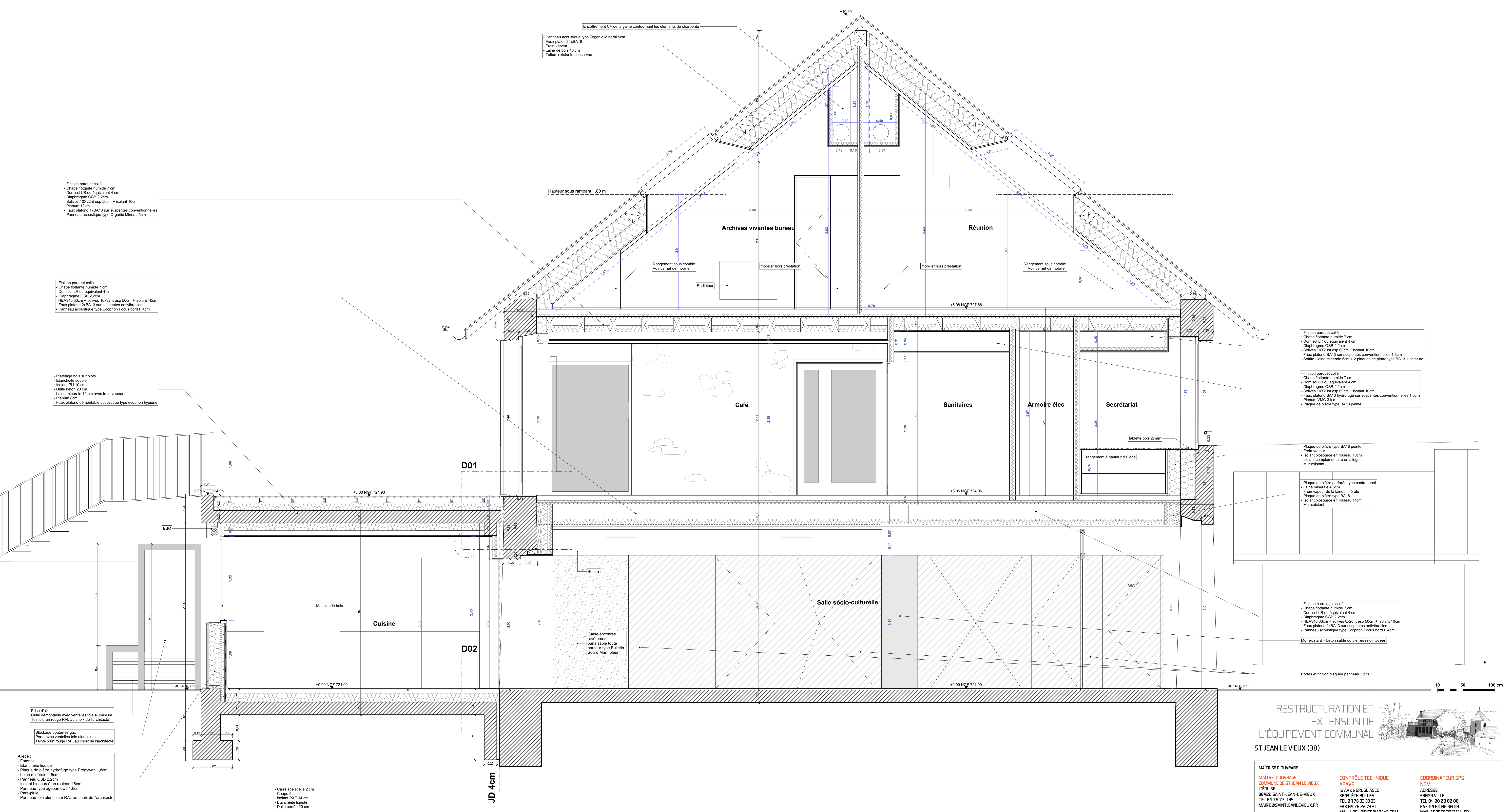
Coupe BB
