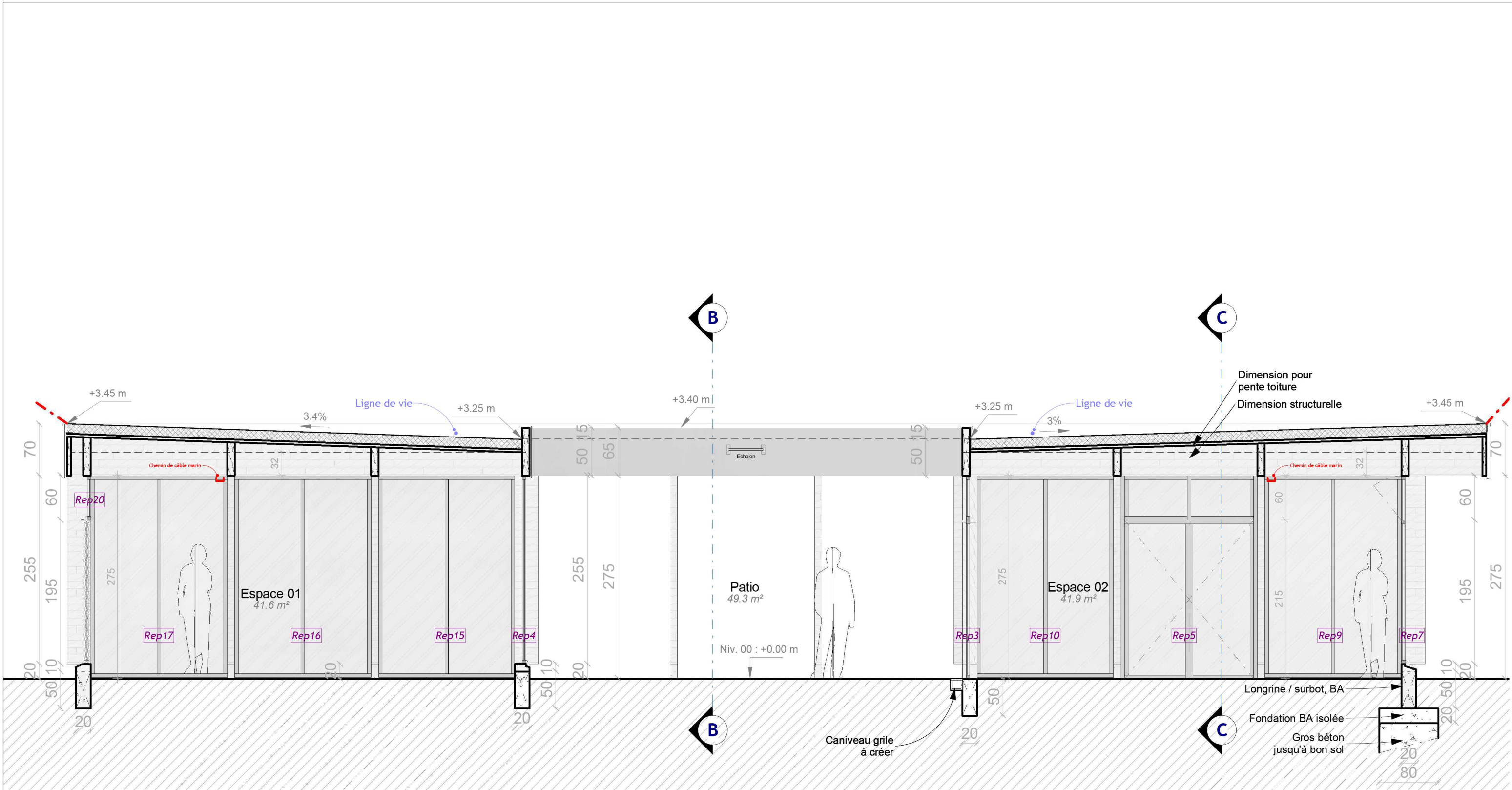
Coupe AA Ech : 1 : 50
