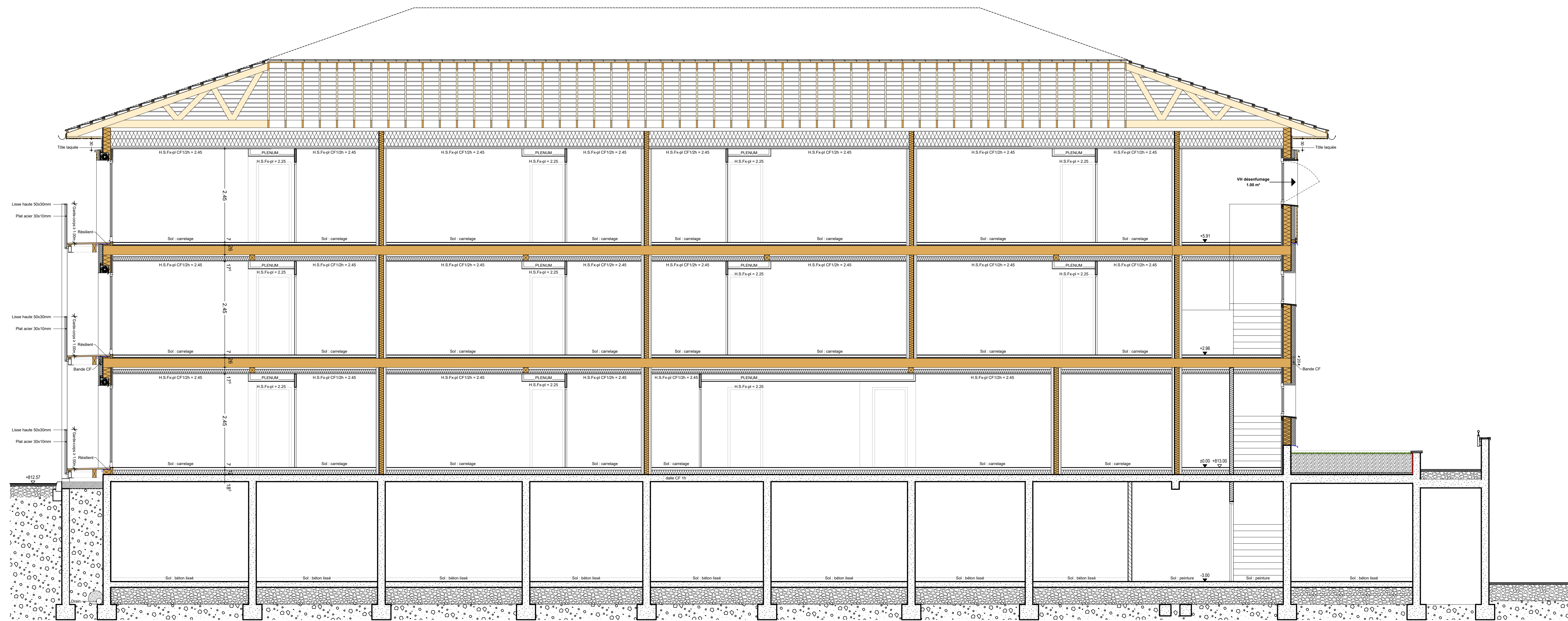
COUPE A2
