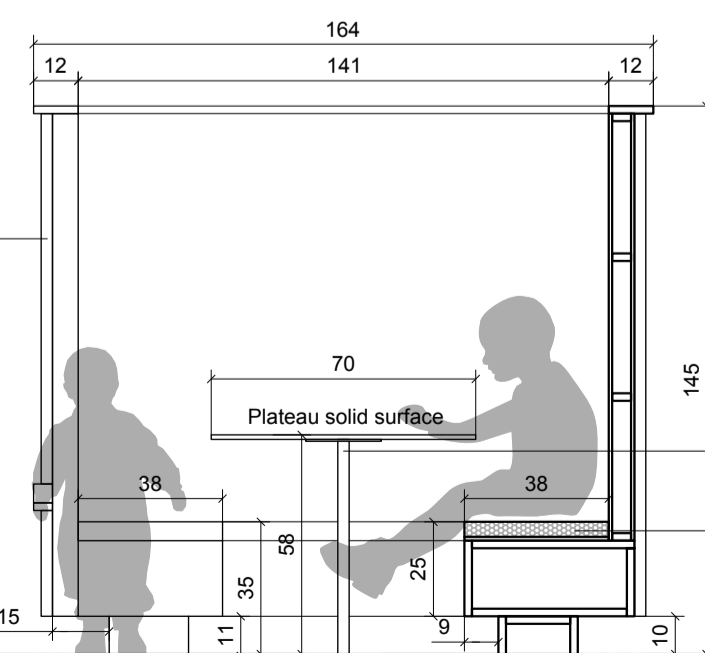
COUPE BB 1/20
