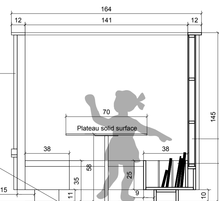
COUPE AA 1/20
