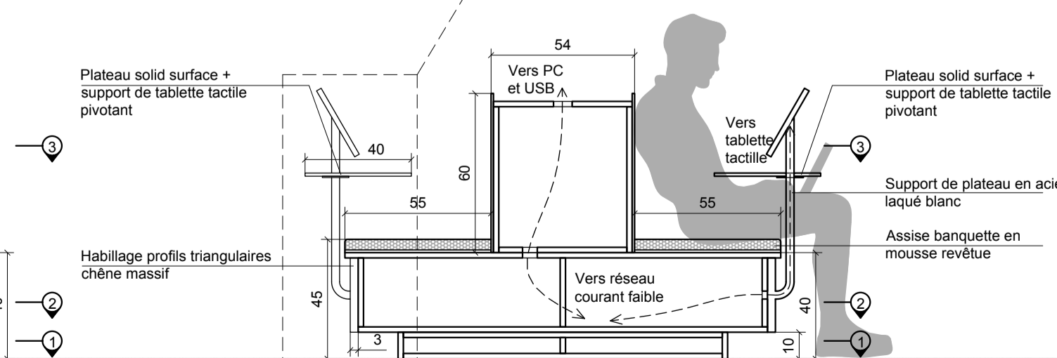
COUPE DD 1/20
