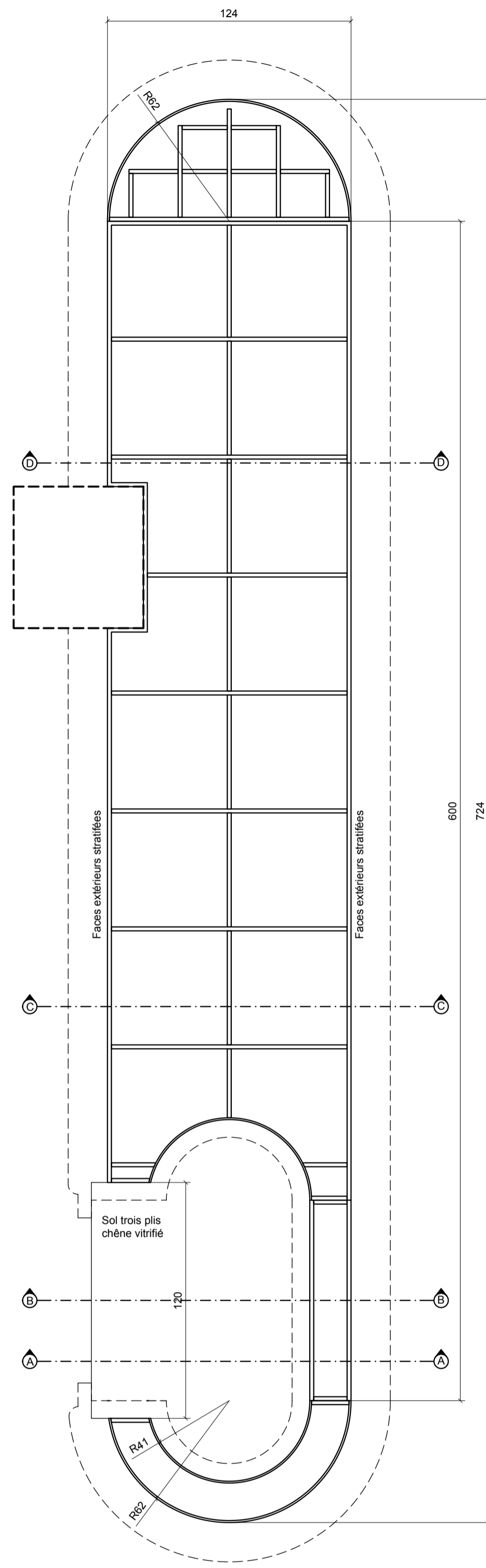
PLAN 1 DANS LE SOCLE 1/20
