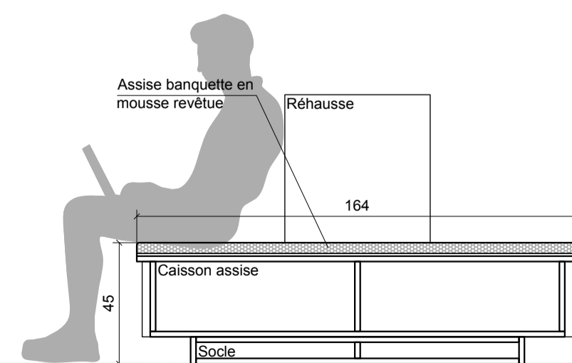
COUPE CC 1/20
