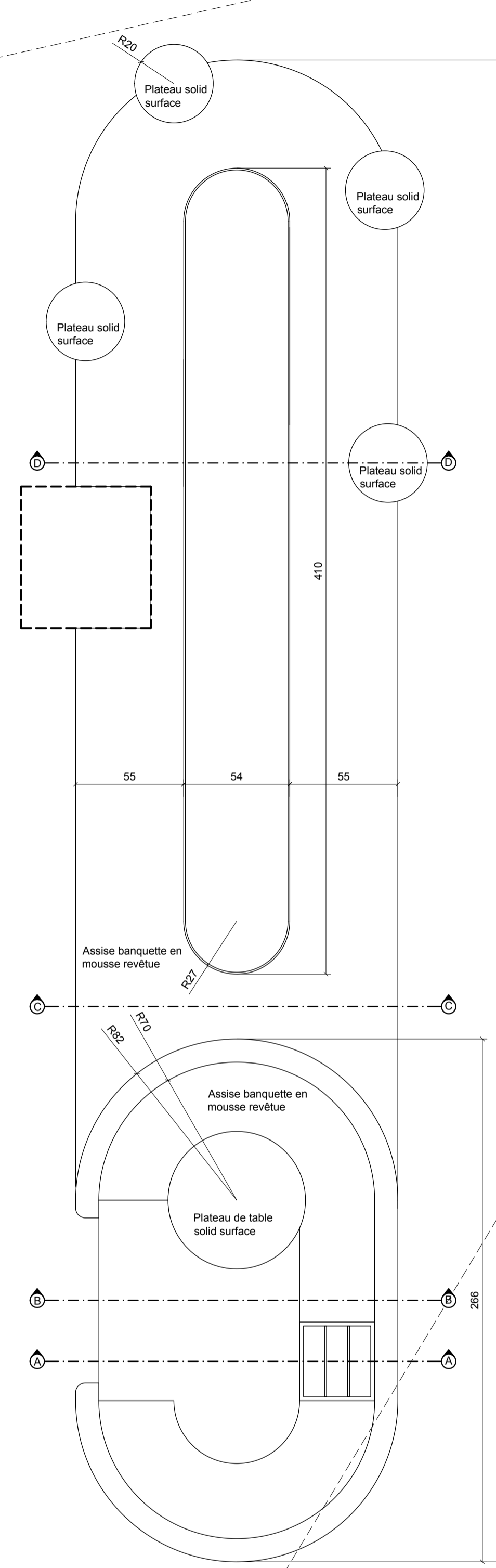
VUE D'ENSEMBLE 1/20
