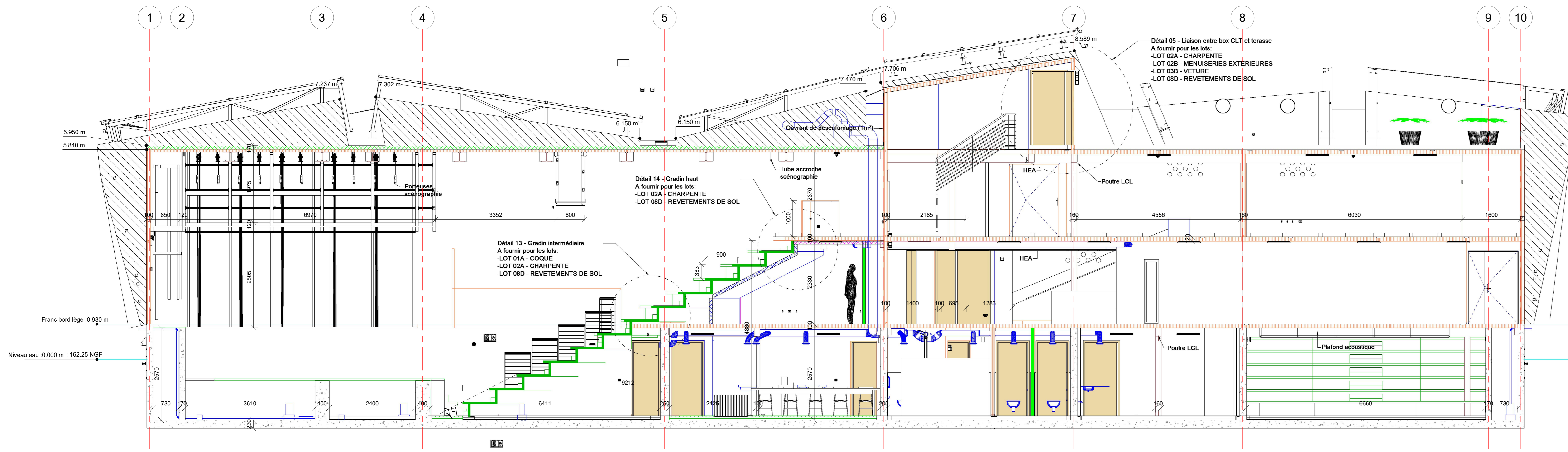
1 COUPE X1 1 : 50
