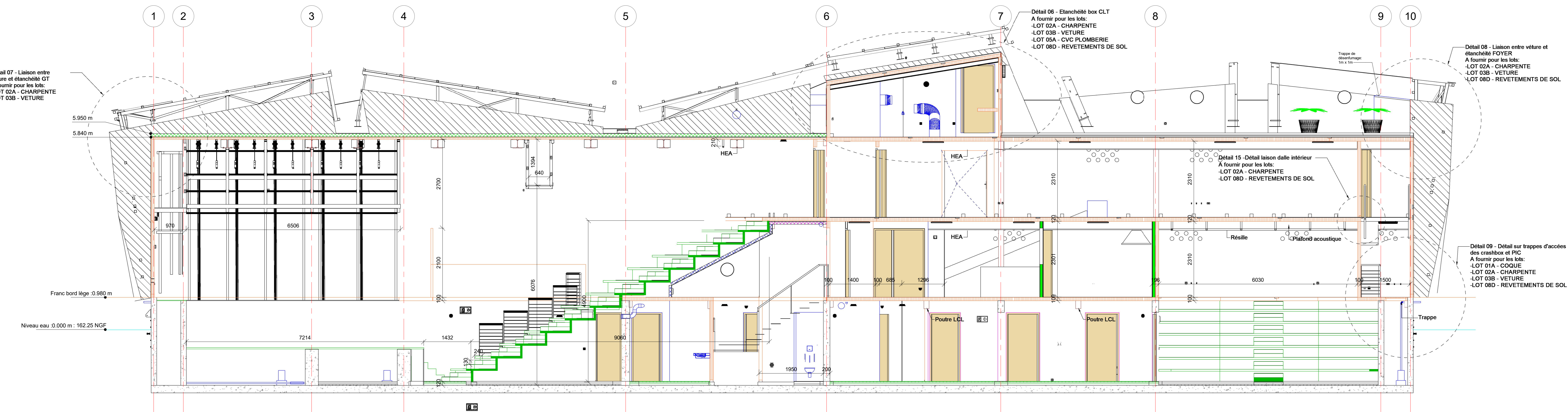
2 COUPE X2 1 : 50
