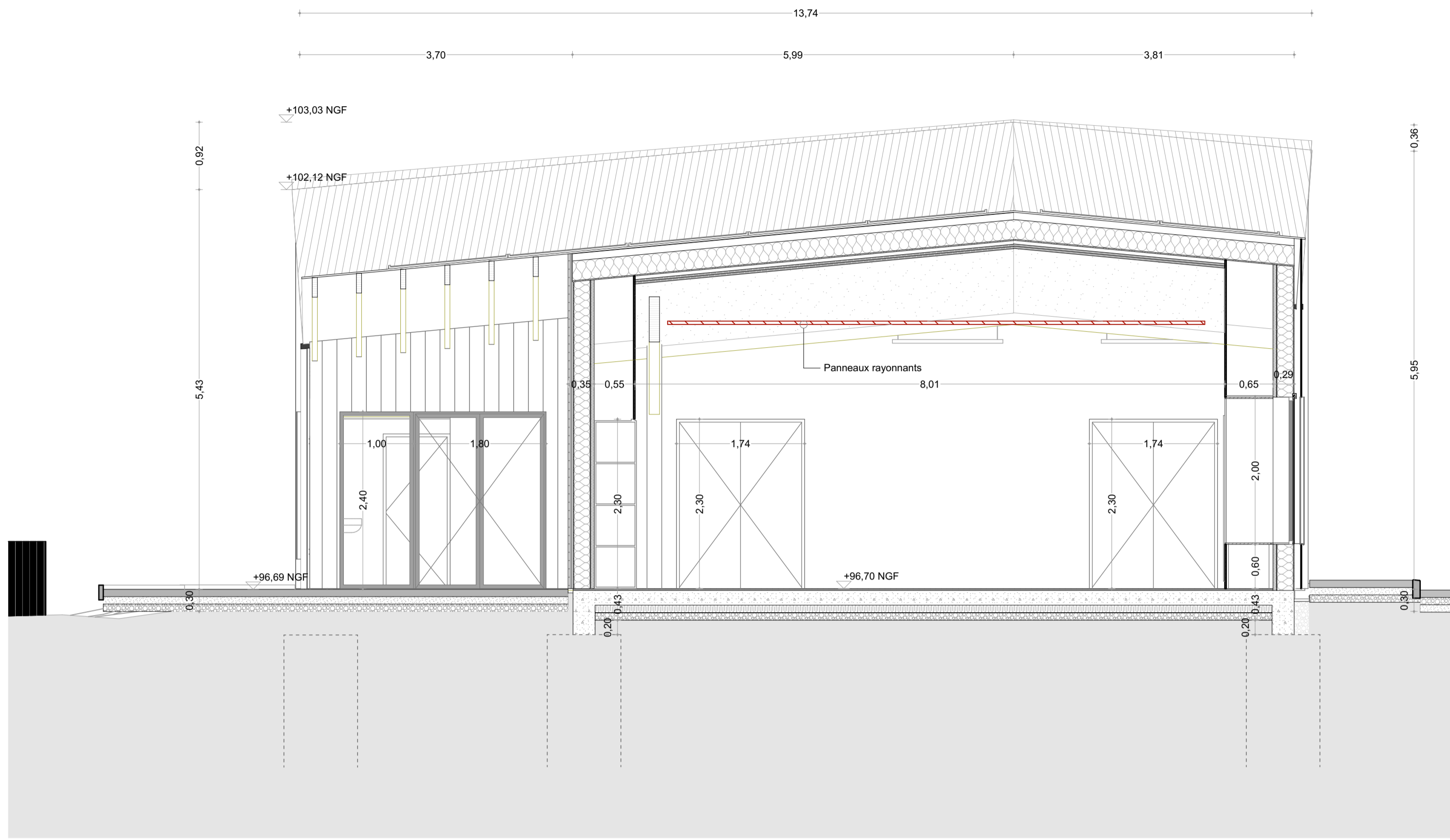
Coupe A
