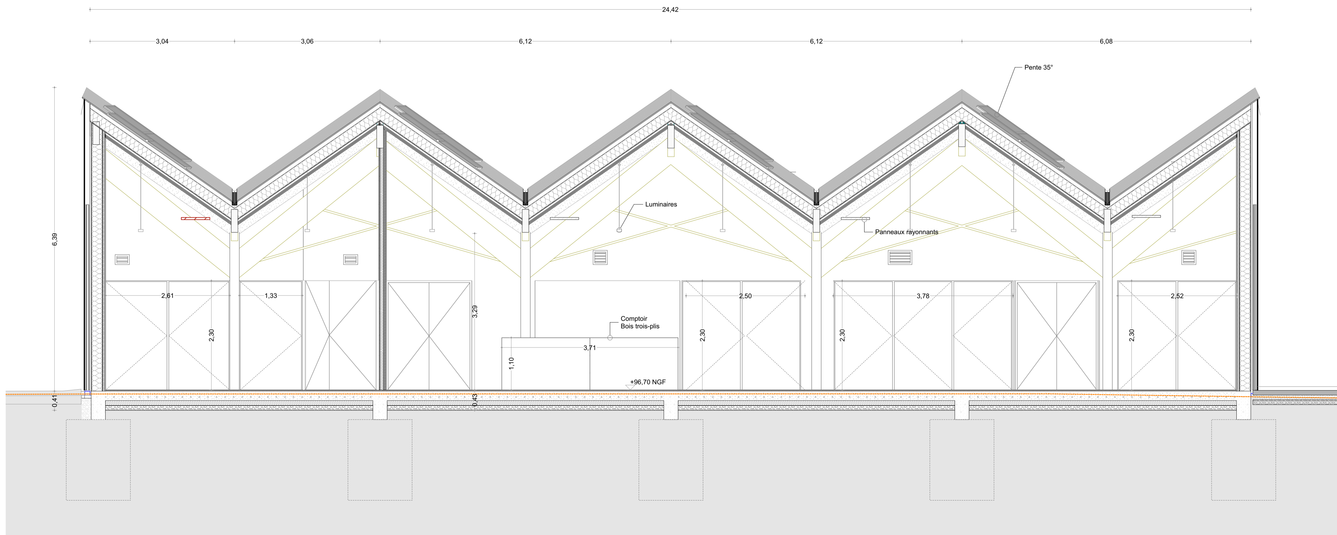
Coupe B
