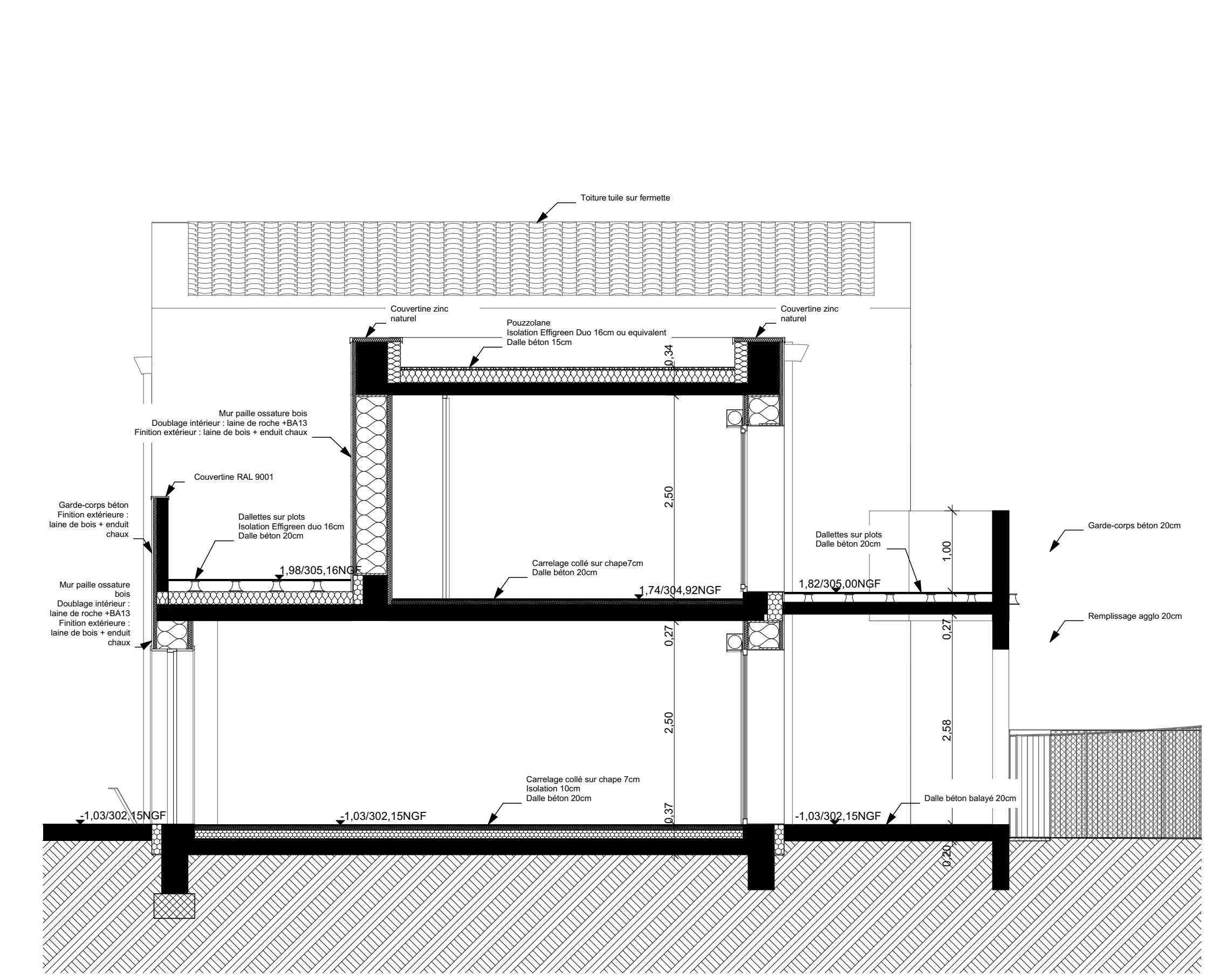
Coupe CC
