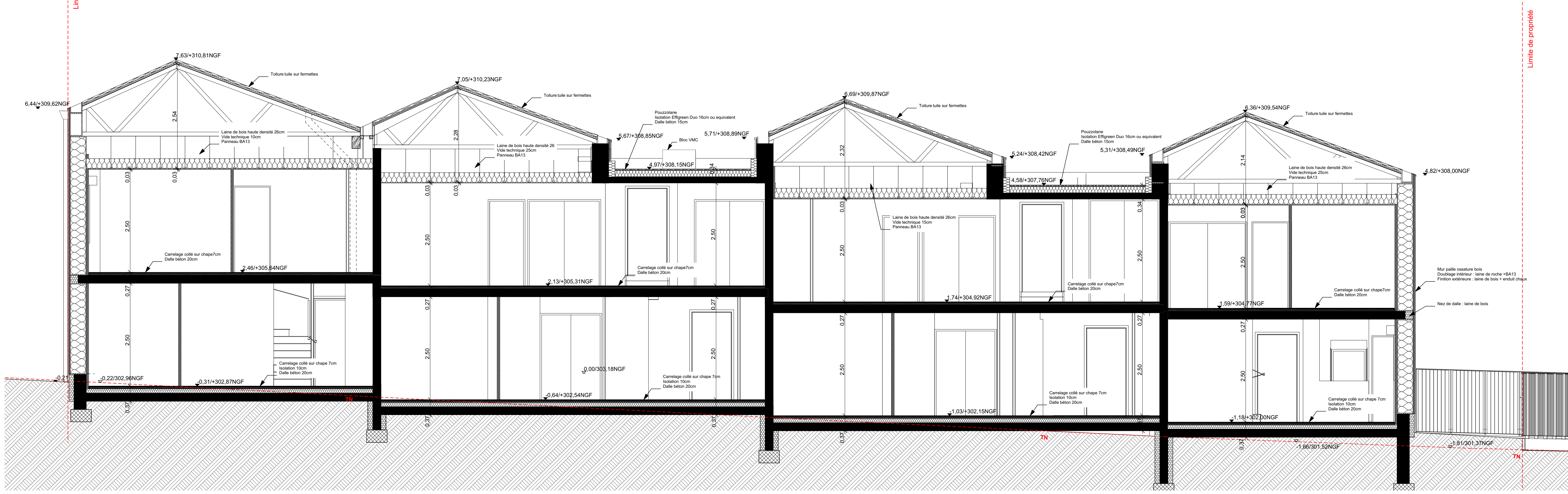
Coupe AA
