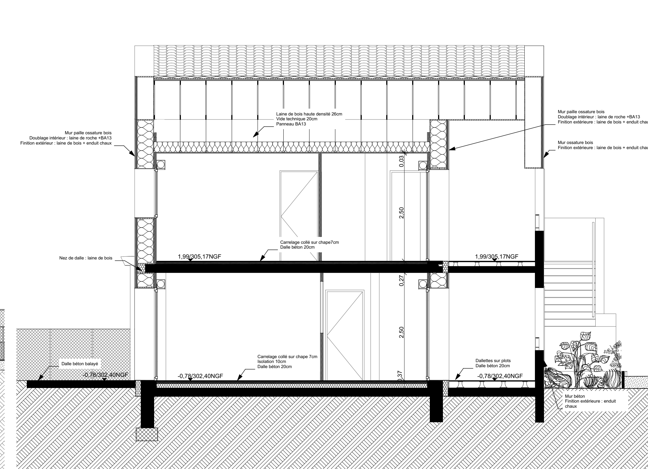
Coupe EE
