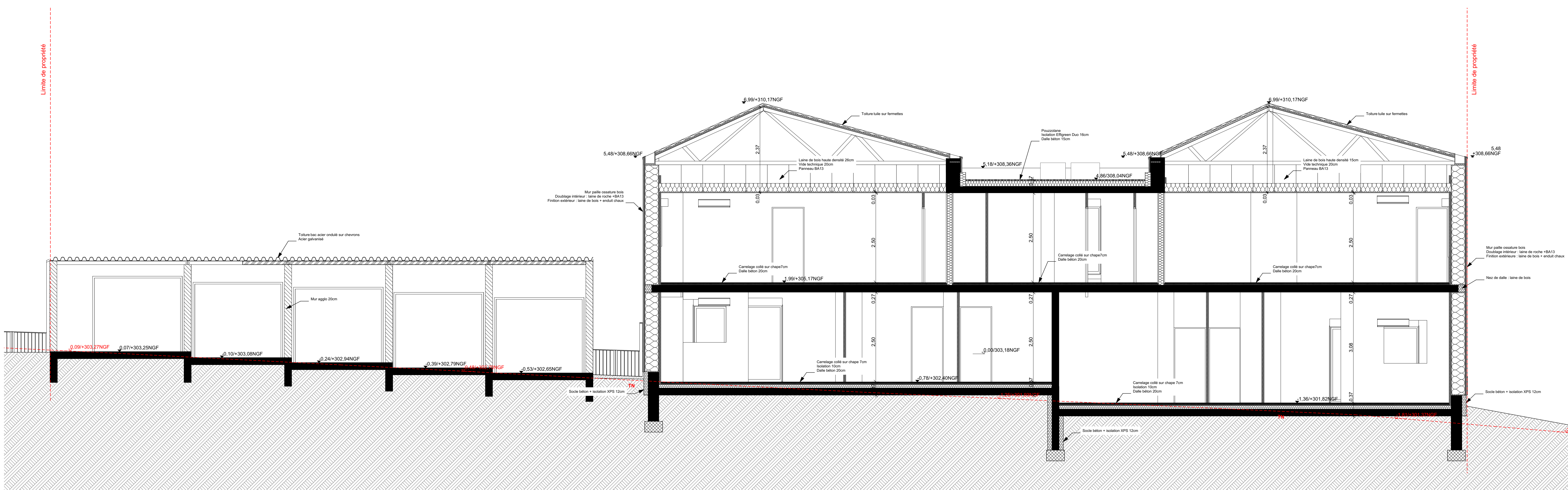
Coupe DD
