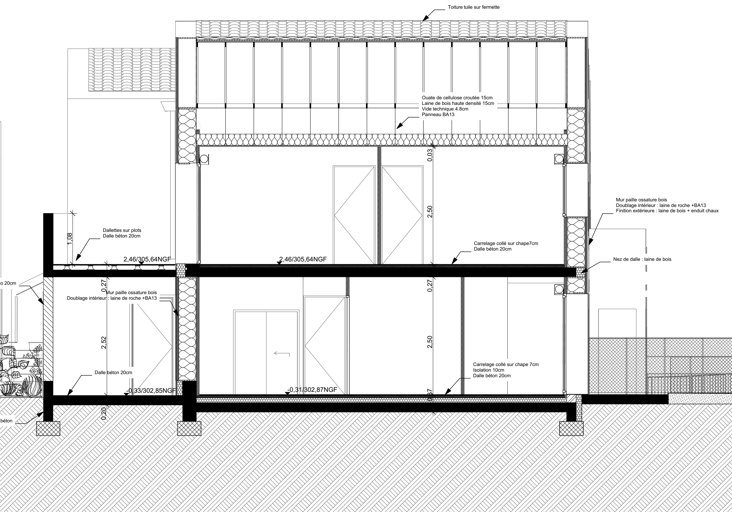
Coupe BB
