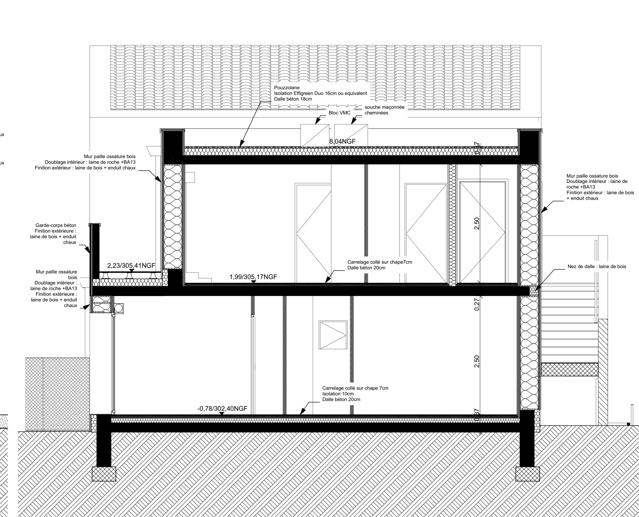
Coupe FF
