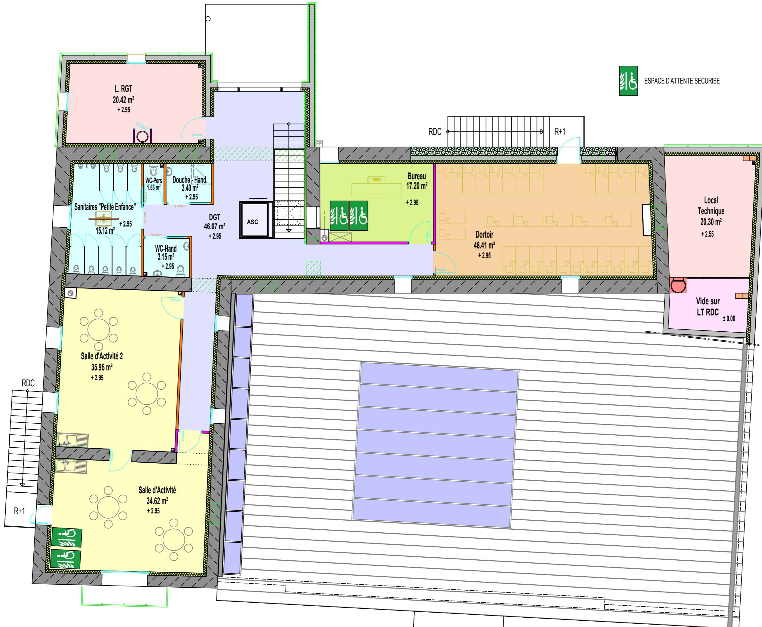
VUE EN PLAN ETAGE - Futur
