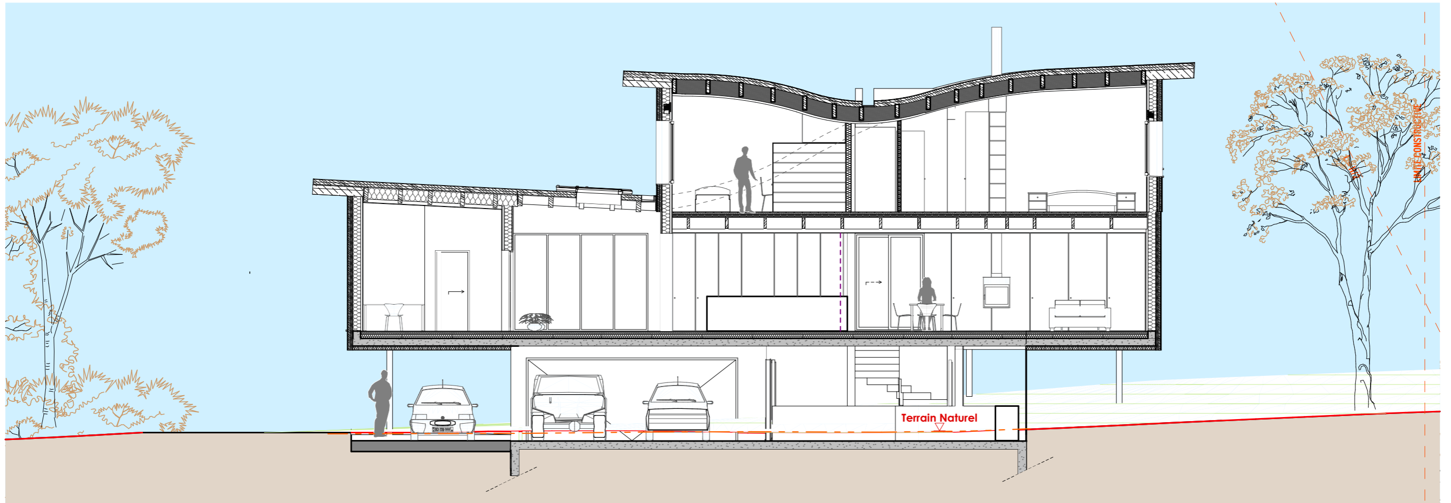
Coupe AA
