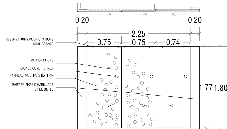
PORTES COULISSANTES SECHOIR & CUMULUS RAILS METALLIQUES A ENCASTRER DANS LE FAUX PLAFOND
