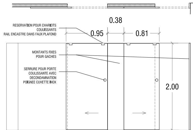
PORTES COULISSANTES SALLE DE BAIN & SALLE D'EAU RAIL METALLIQUE A ENCASTRER DANS LE FAUX PLAFOND
