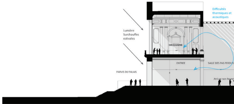
COUPE EXISTANTE
