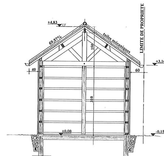
COUPE TRANSVERSALE SUR GARAGE
