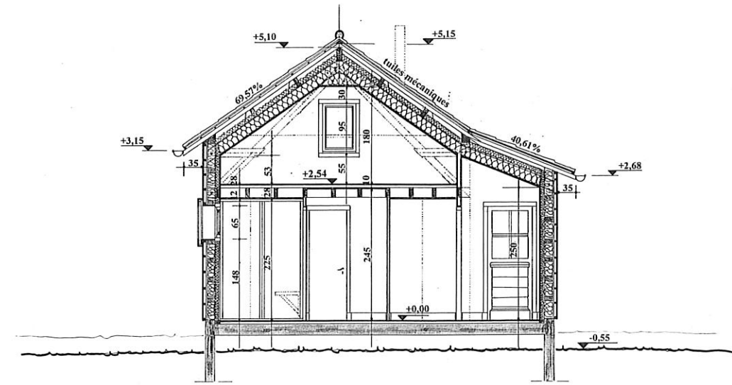
COUPE TRANSVERSALE SUR ANNEXE MAISON D'HABITATION
