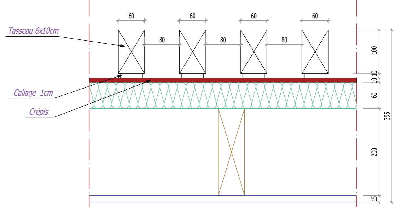
Détails bardage façade Nord
