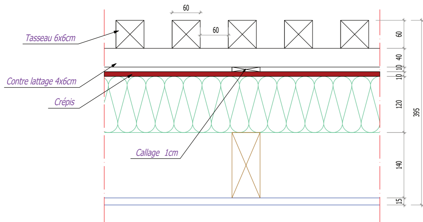
Détails bardage sur lucarne
