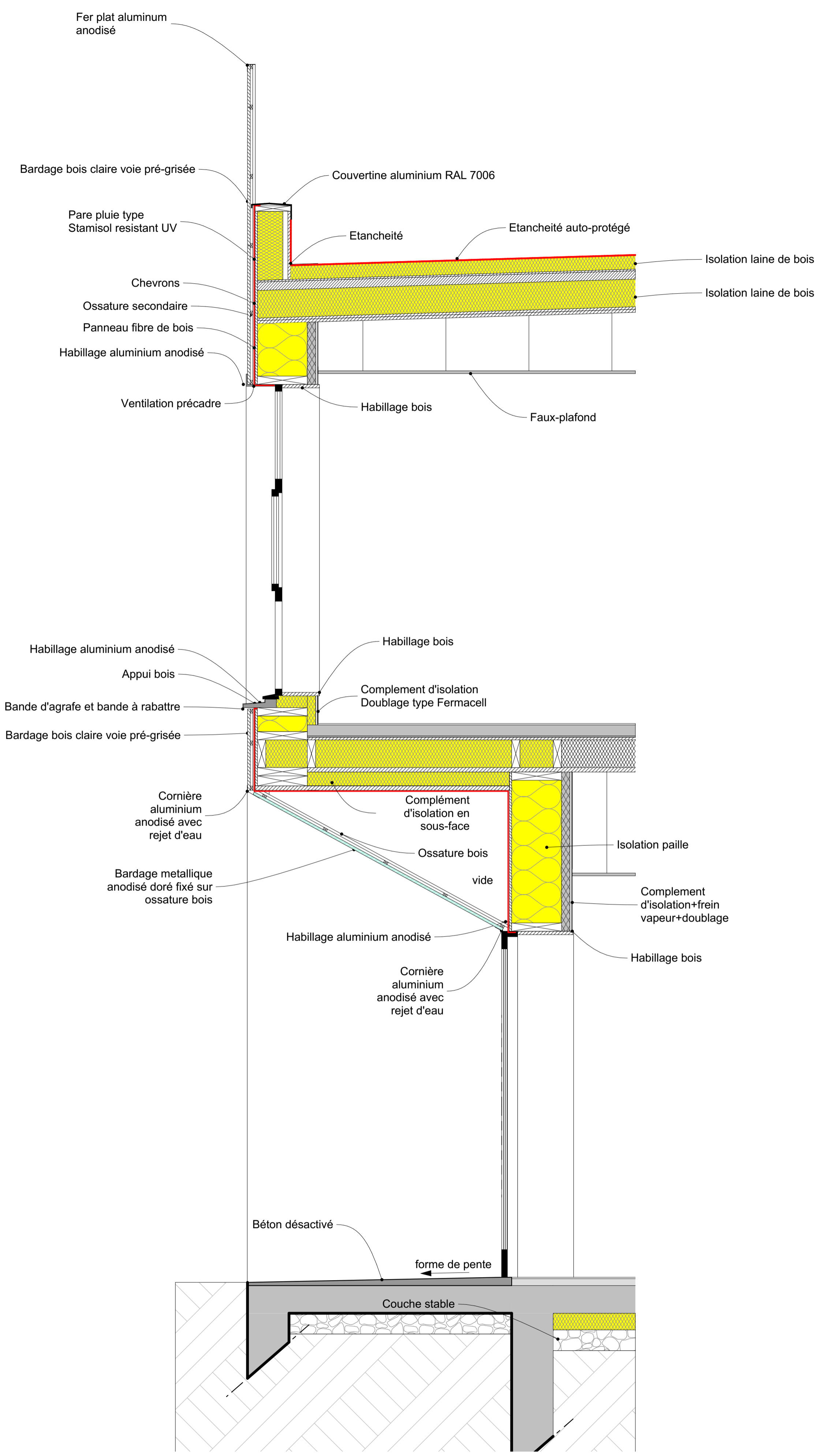
Détails ossature bois porche
