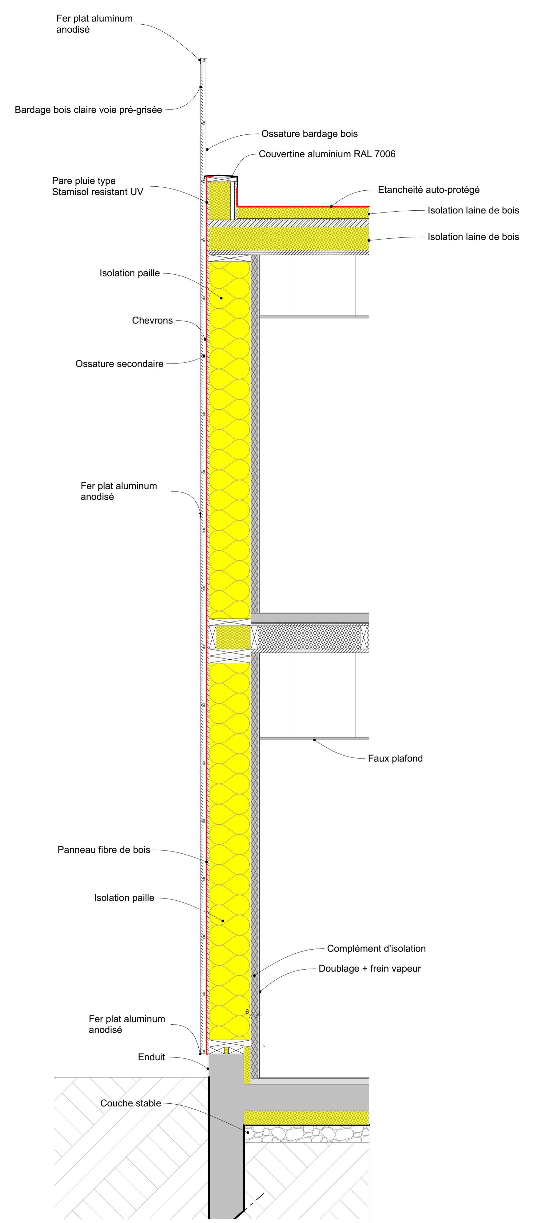
Détails ossature bois murs courants
