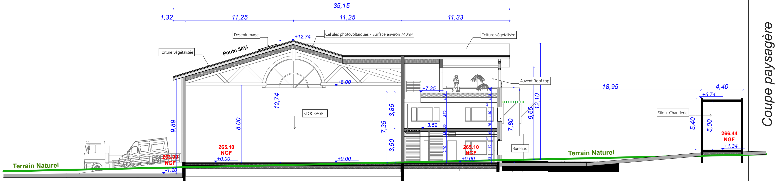
COUPE DE PRINCIPE
