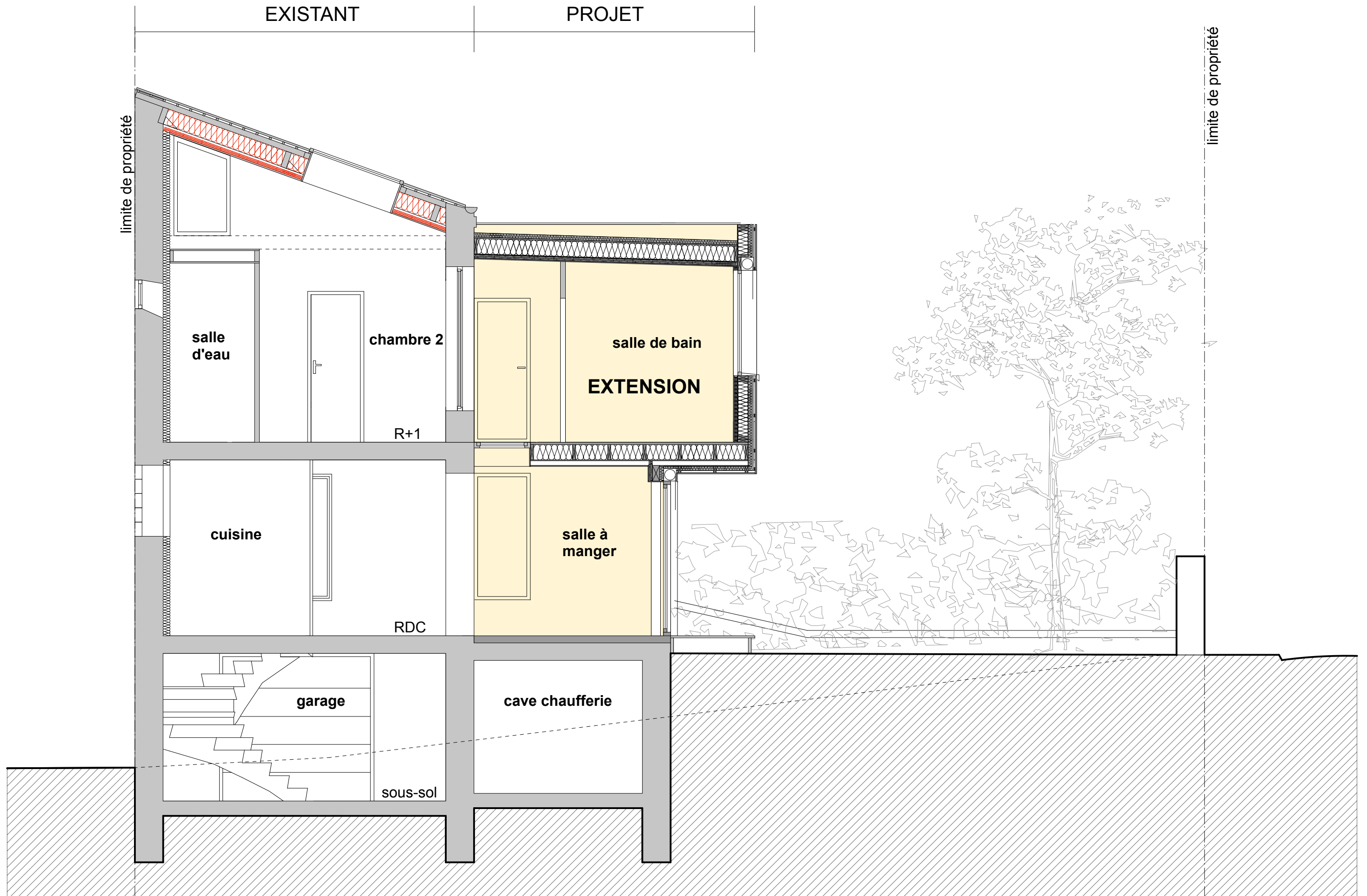
COUPE AA PROJET 1/50e
