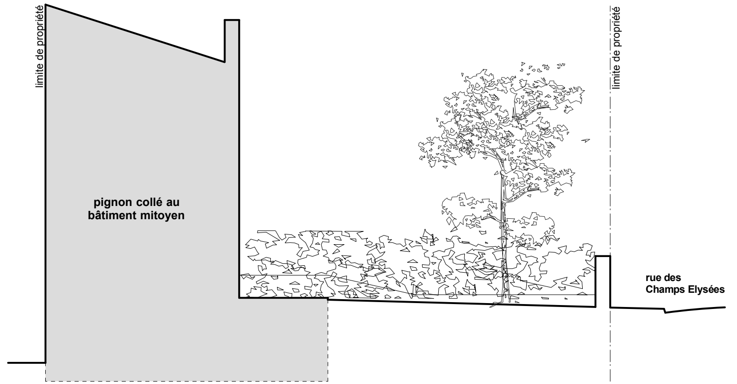
PIGNON NORD EST, CONTRE LE BATIMENT MITOYEN
