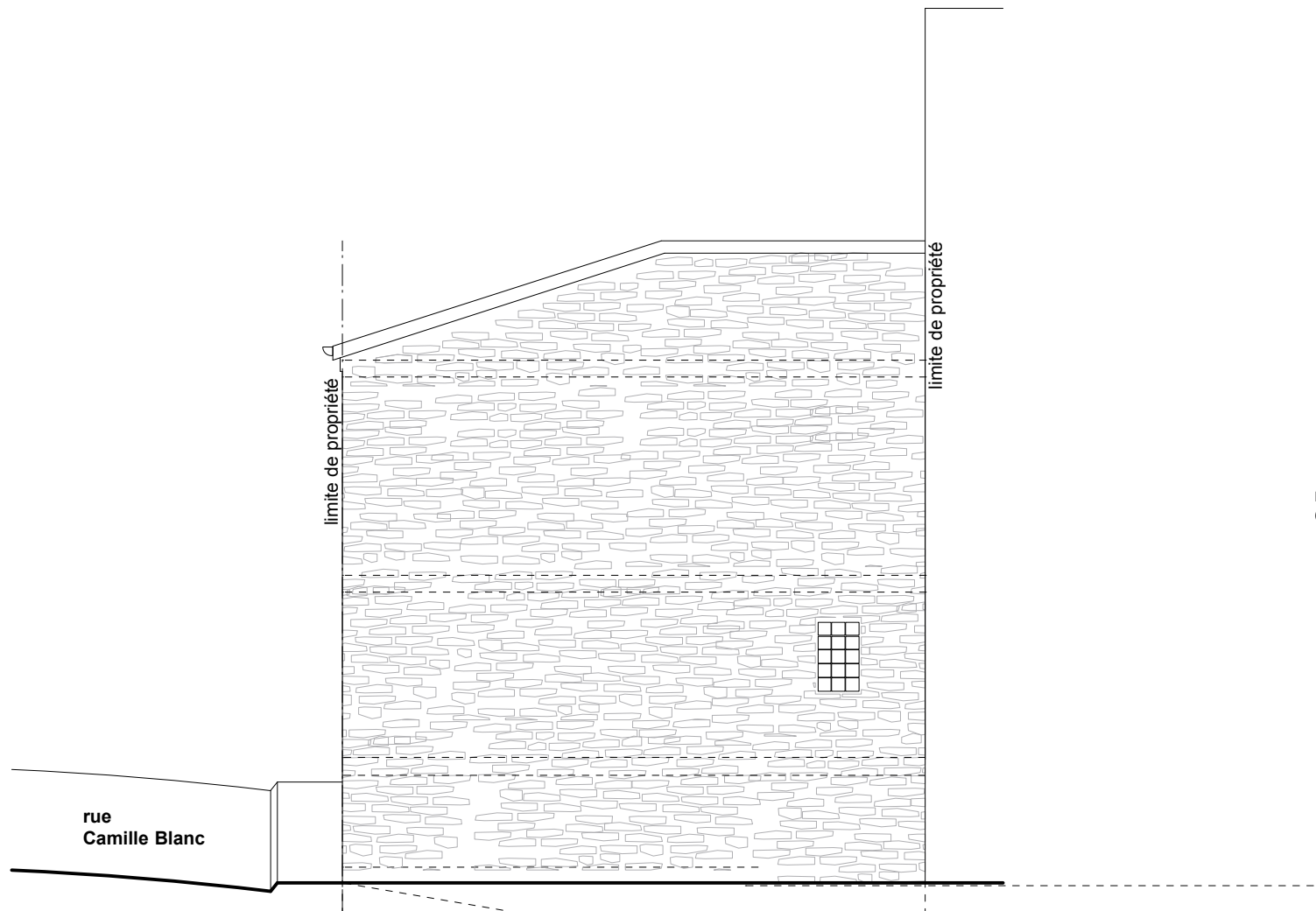
PIGNON SUD EST, EN LIMITE DE PROPRIETE
