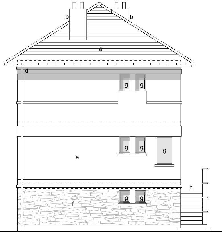
FACADE EST
