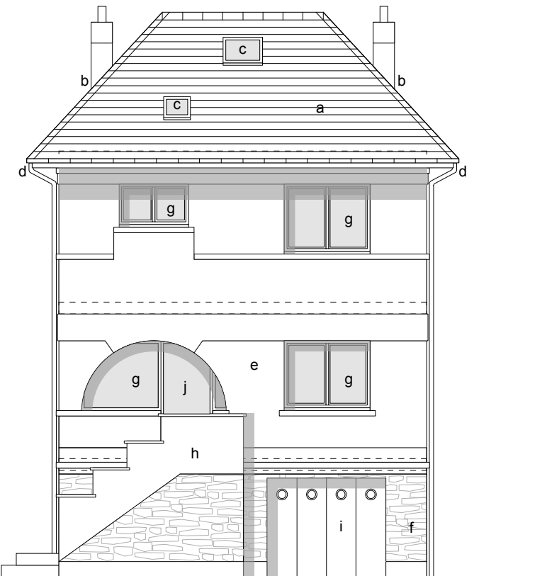
FACADE NORD RUE sans clôture
