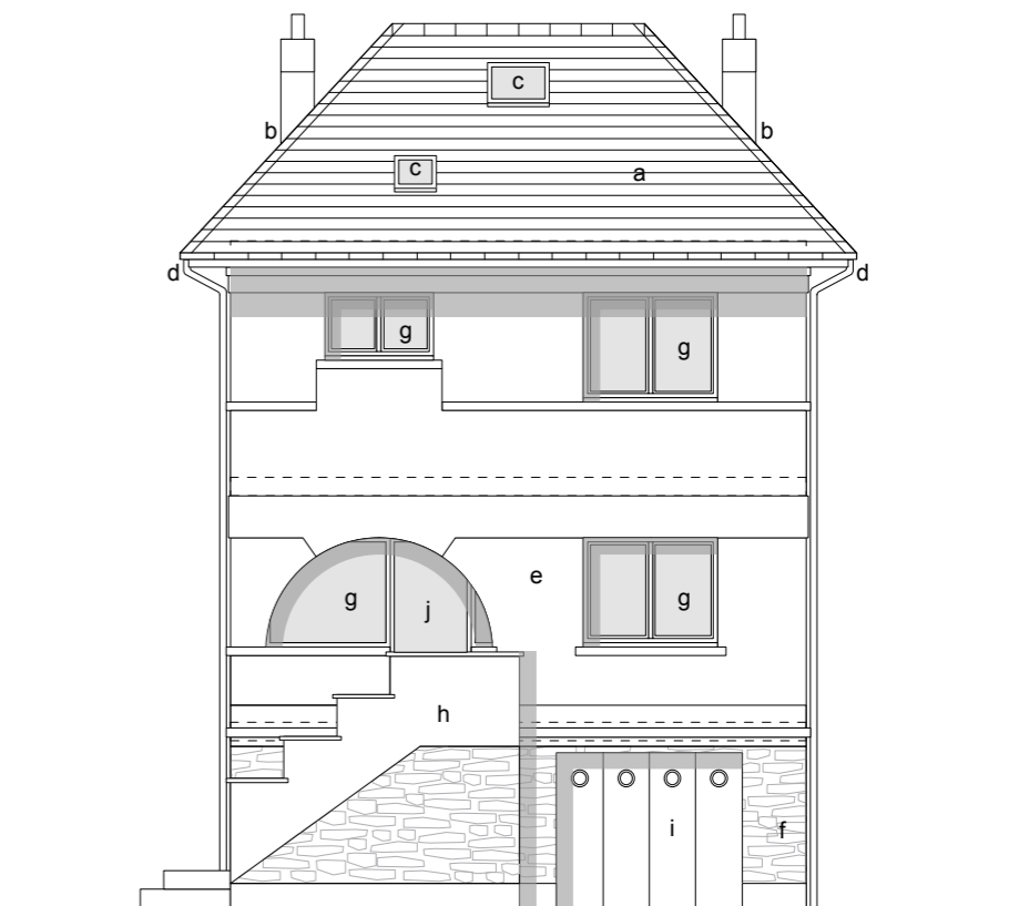
FACADE NORD RUE sans clôture
