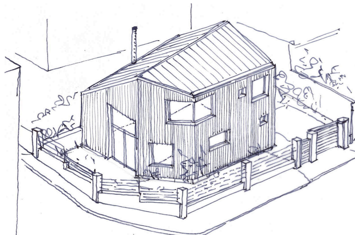
axonométrie angle rue Offenbach et voie Verdi
