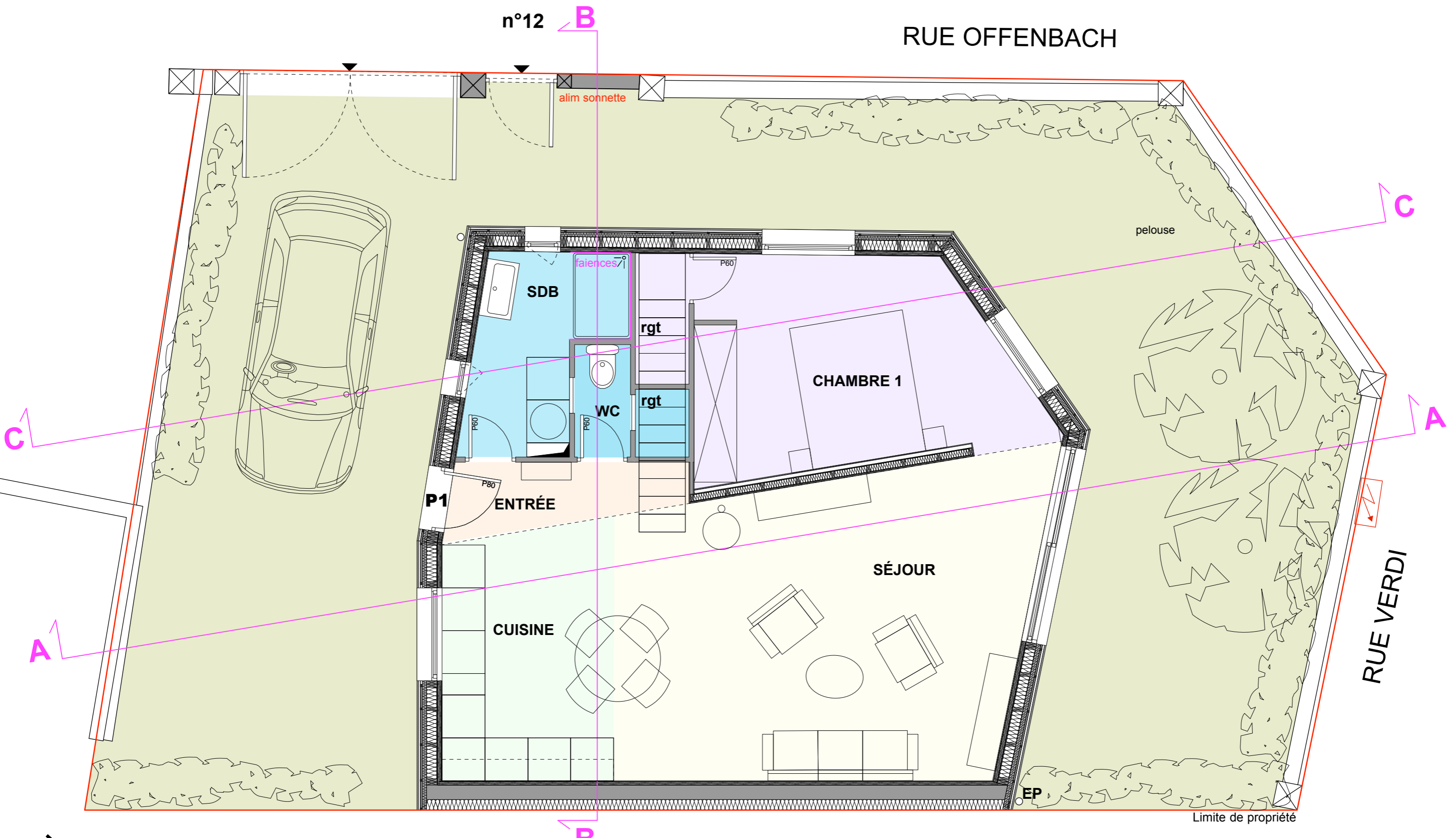
PLAN RDC
