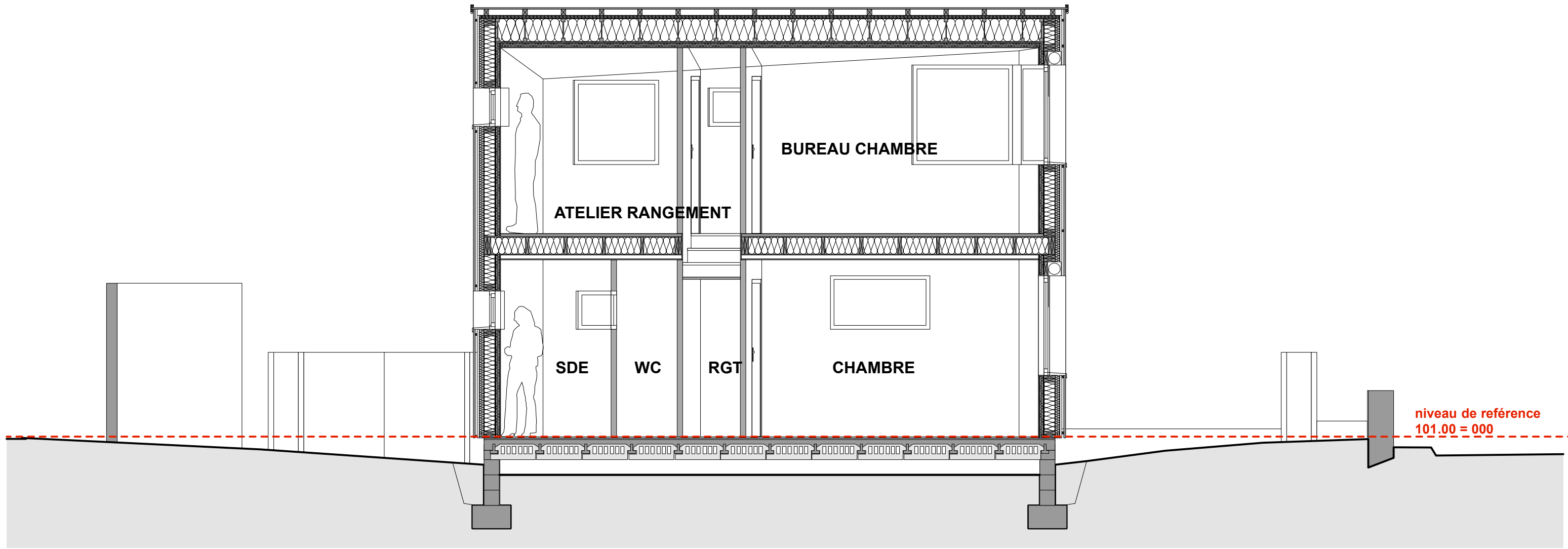
COUPE LONGITUDINALE CC 1/50e
