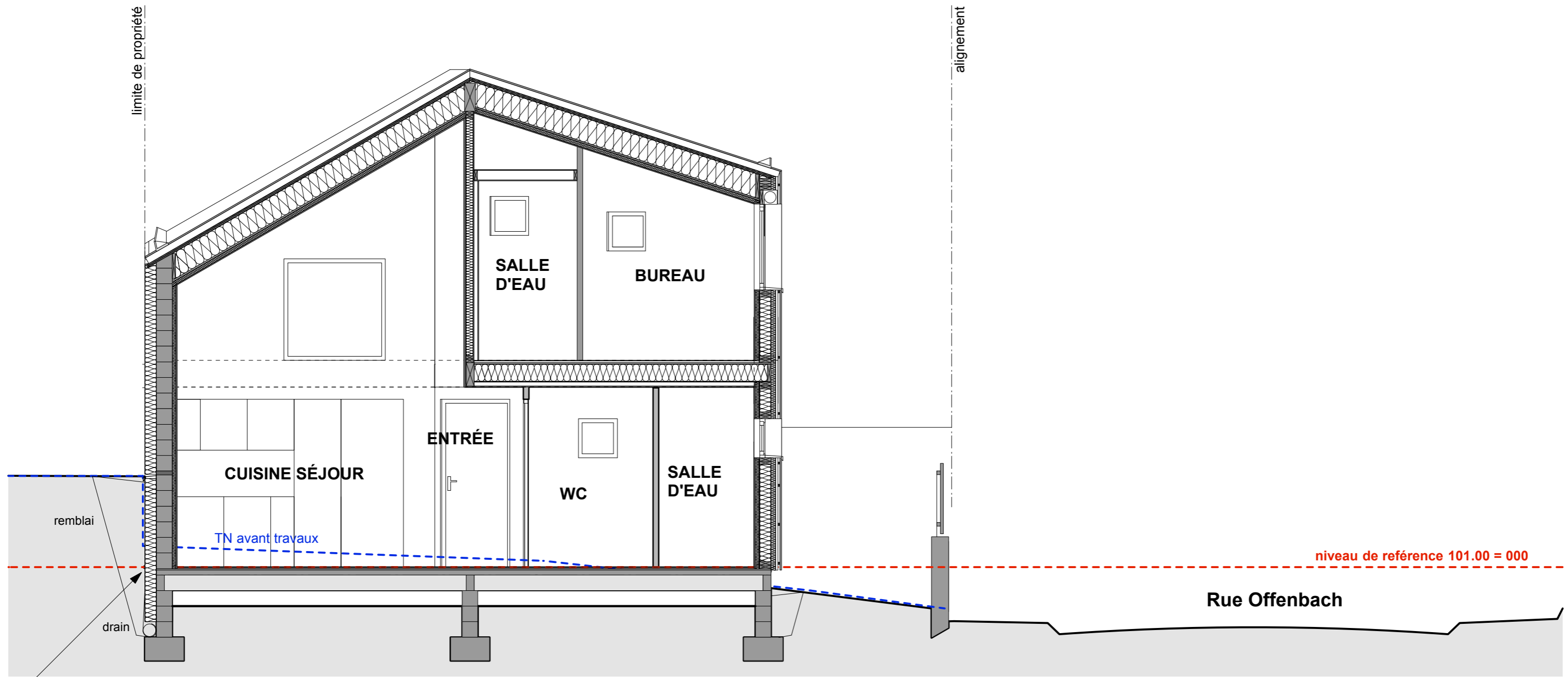
COUPE TRANSVERSALE BB 1/50e
