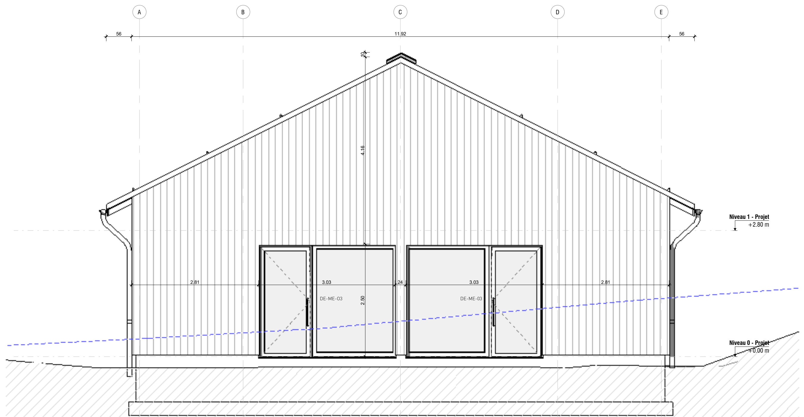
FA-02 - Façade
