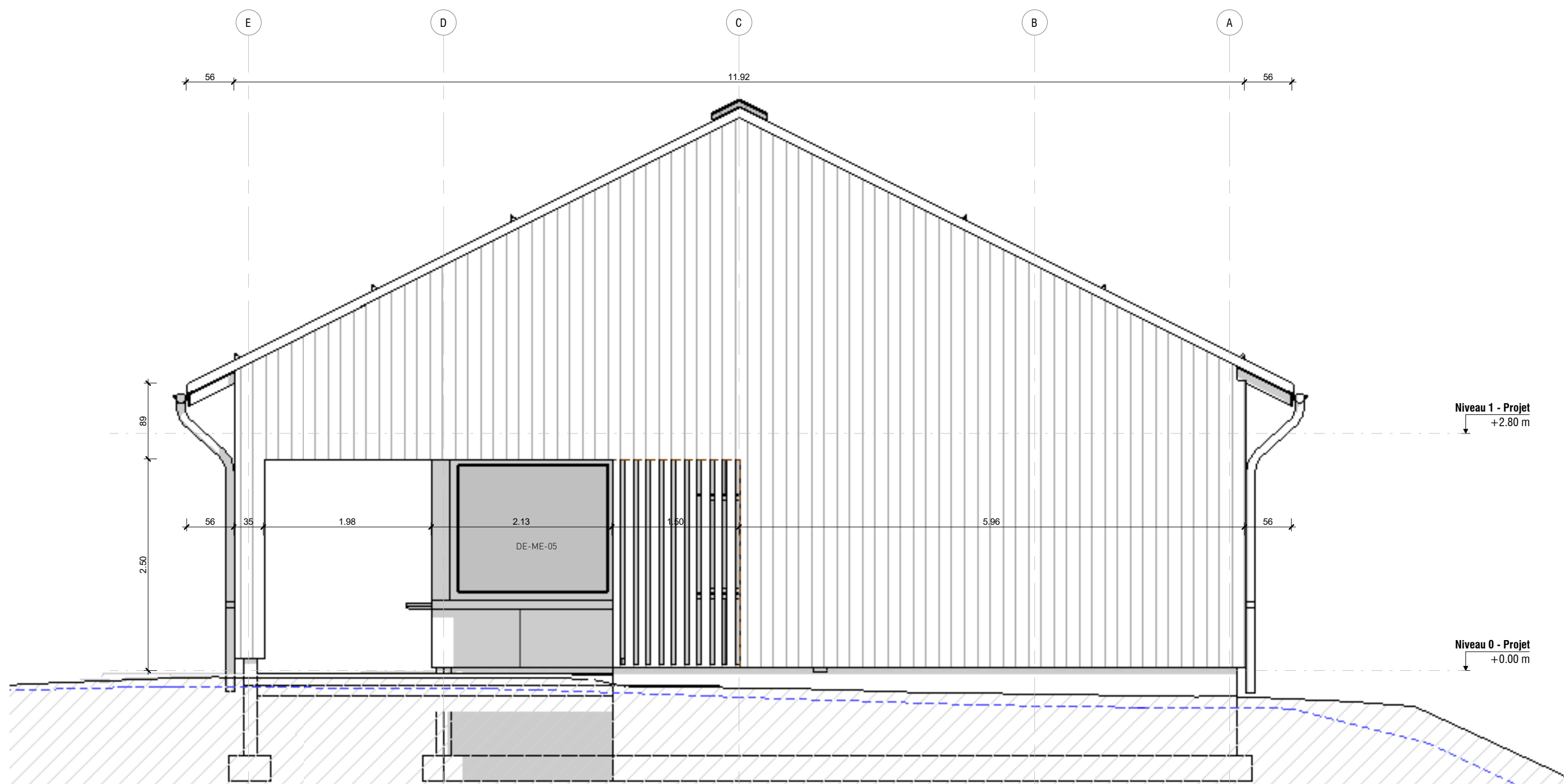
FA-01 - Façade
