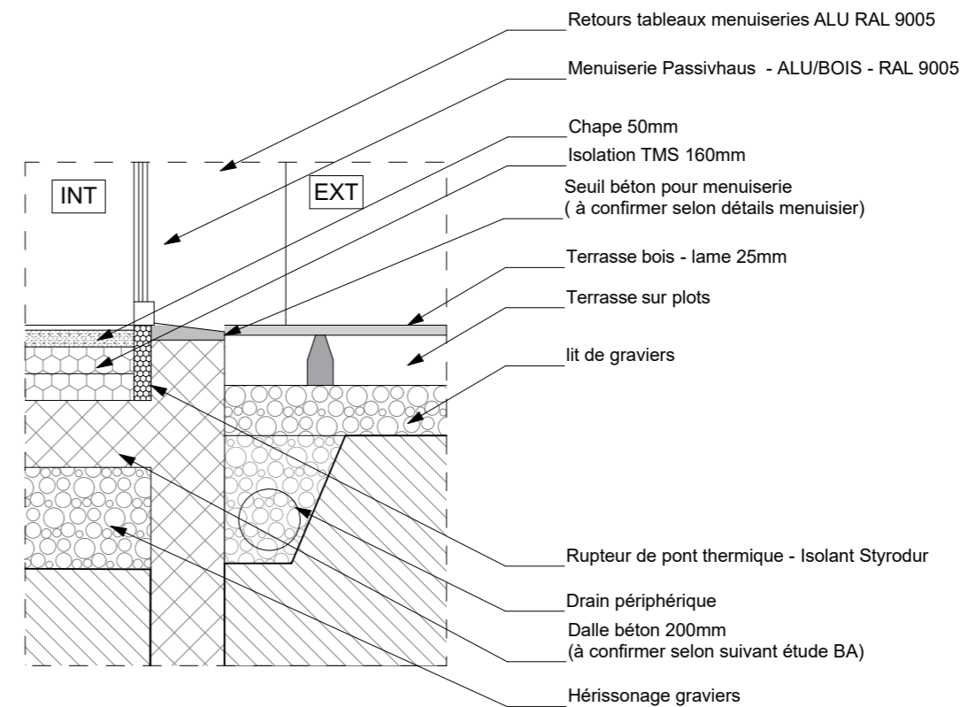
DÉTAIL 07 / Dalle 3 : Seuil vers terrasse
