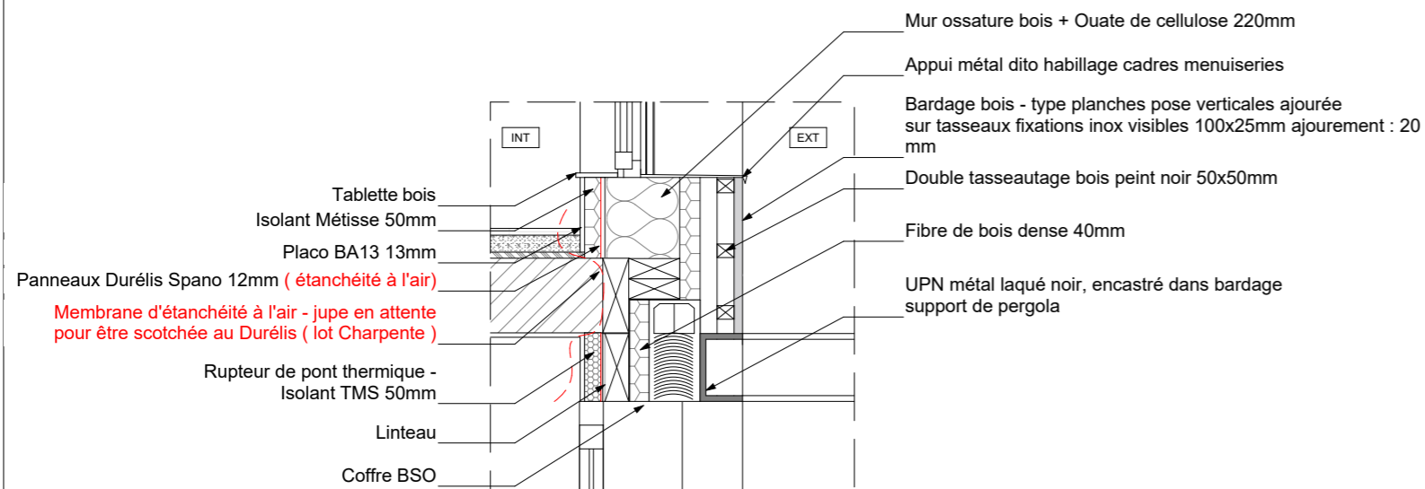
DÉTAIL 08 / Dalle 4 : BSO / UPN pergola
