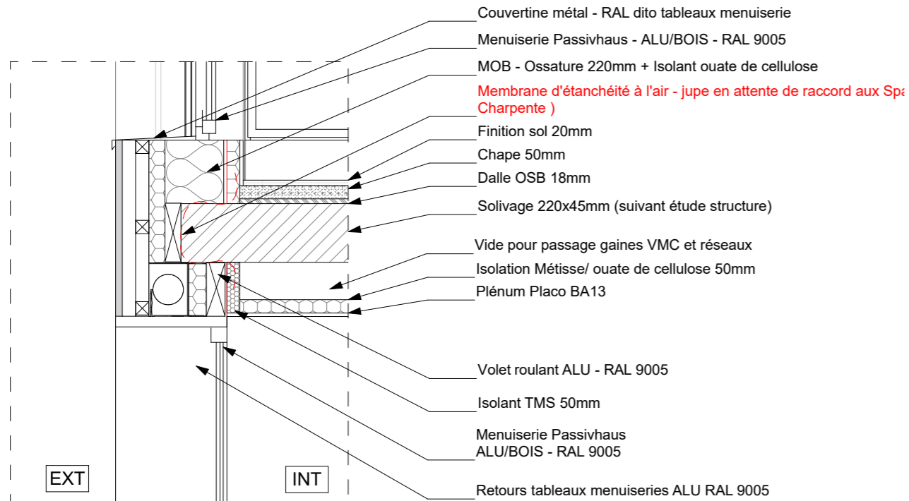
DÉTAIL 06 / Dalle 2 : Jonction MOB et plancher R+1
