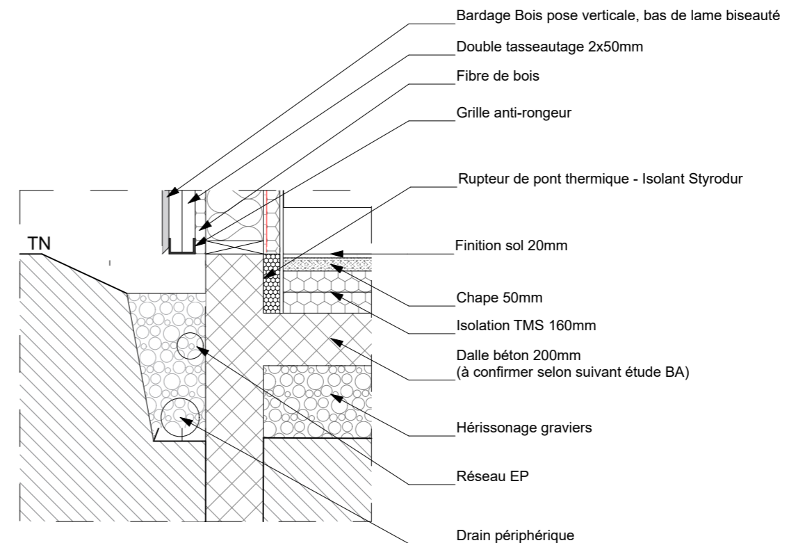
DÉTAIL 09 / Dalle 1 : mur/dalle façade NORD
