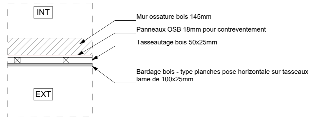
DÉTAIL 03 / Mur 3 : Mur annexe MOB 145mm
