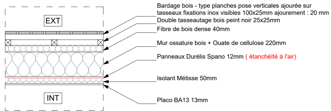
DÉTAIL 01 / Mur 1 : Mur maison MOB 220mm
