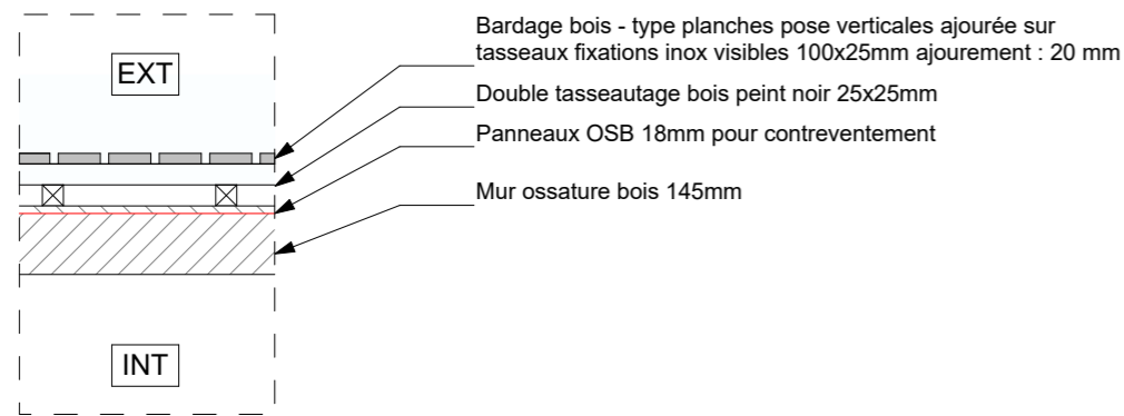
DÉTAIL 02 / Mur 2 : Mur garage MOB 145mm
