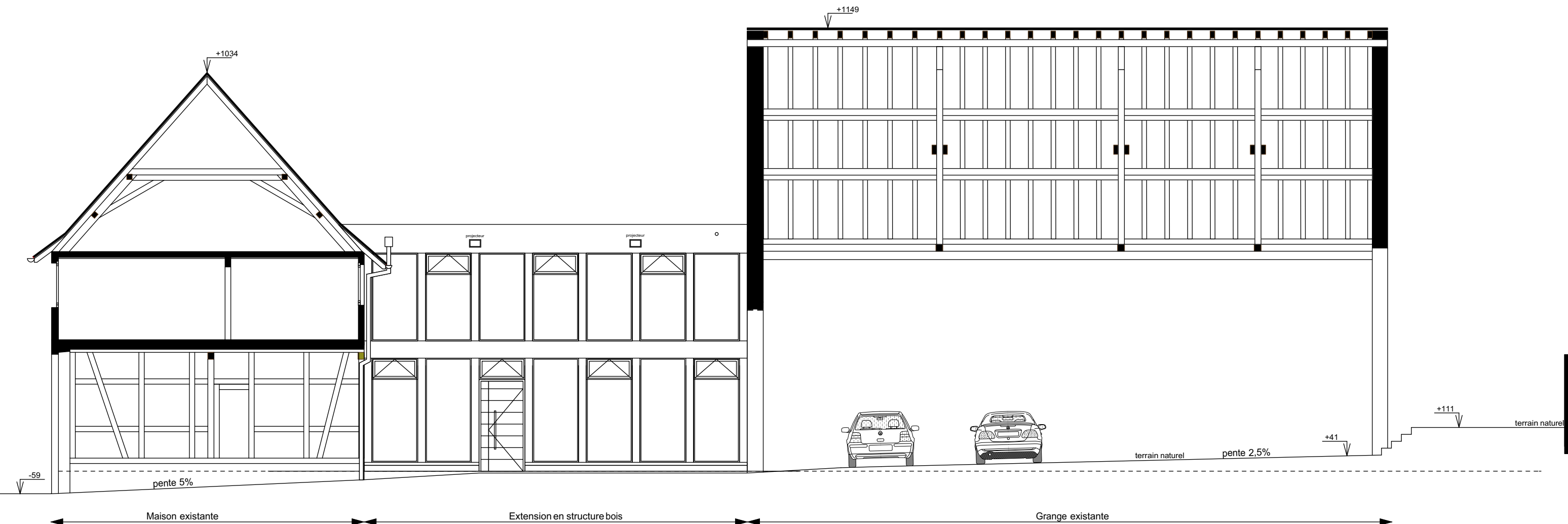
COUPE / FACADE NORD FF
