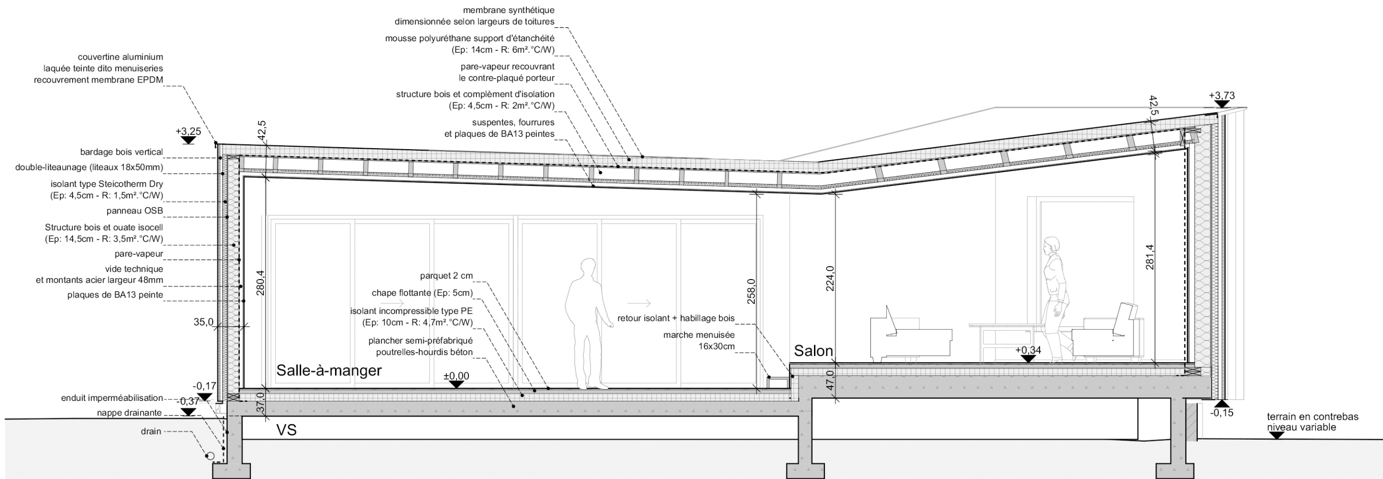
Coupe AA - séjour-salon
