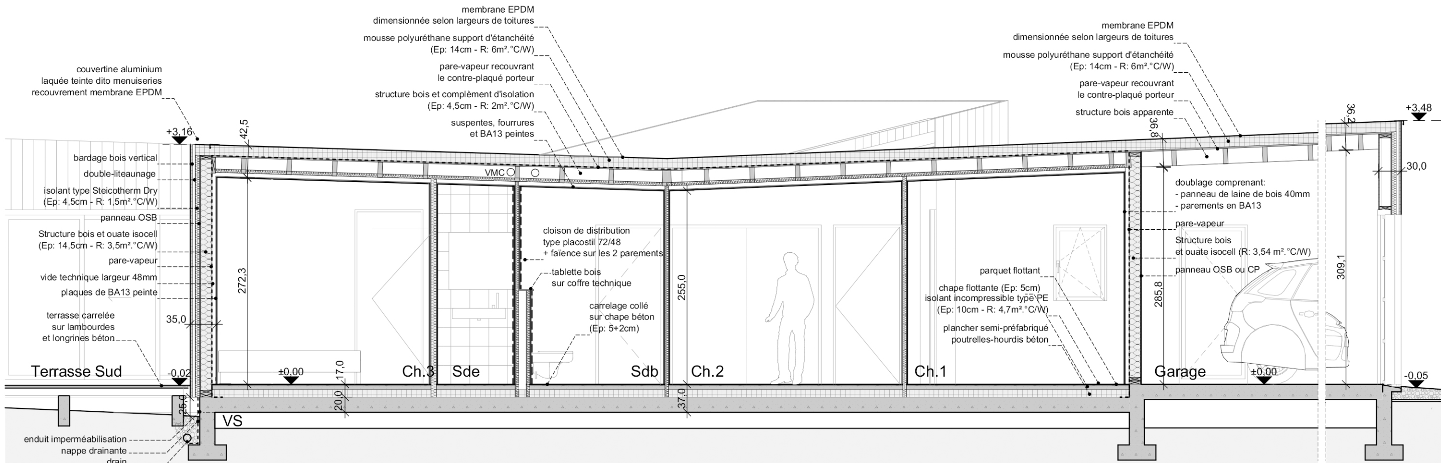
Coupe BB - zone nuit et garage
