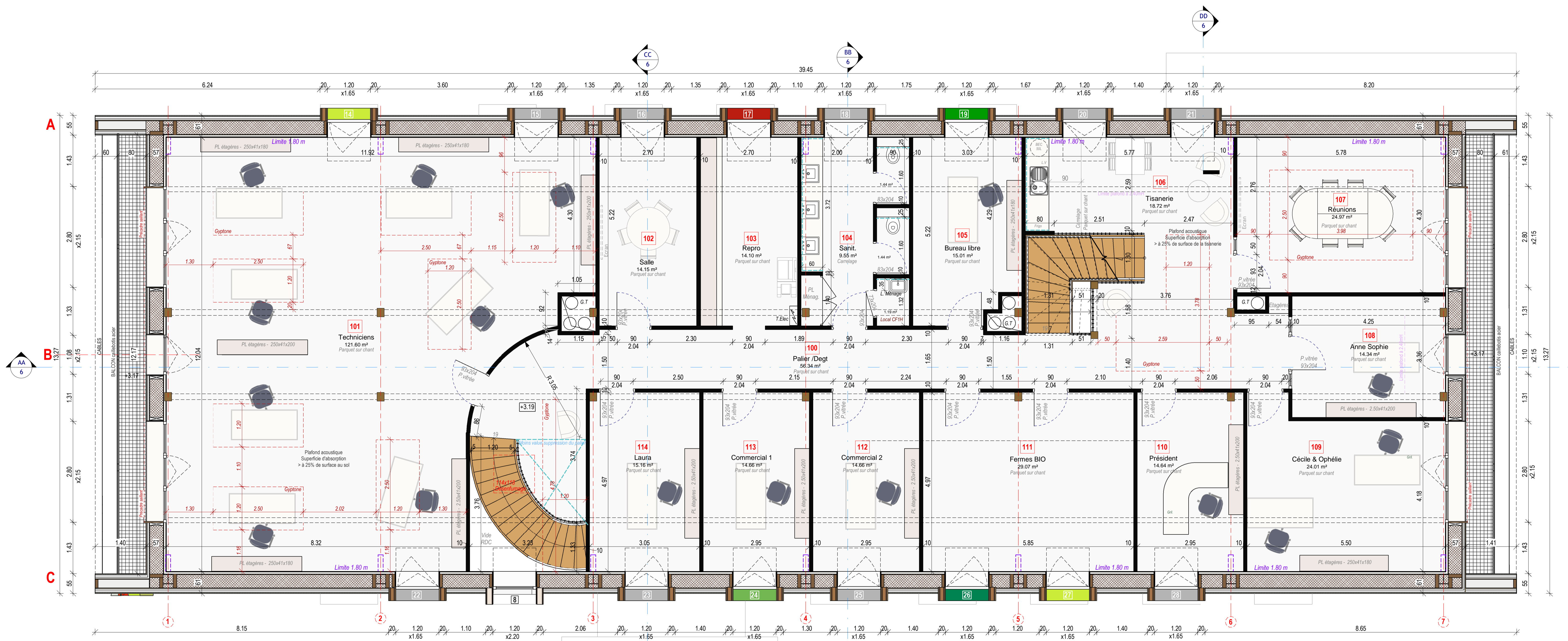
Combles 1 : 50
