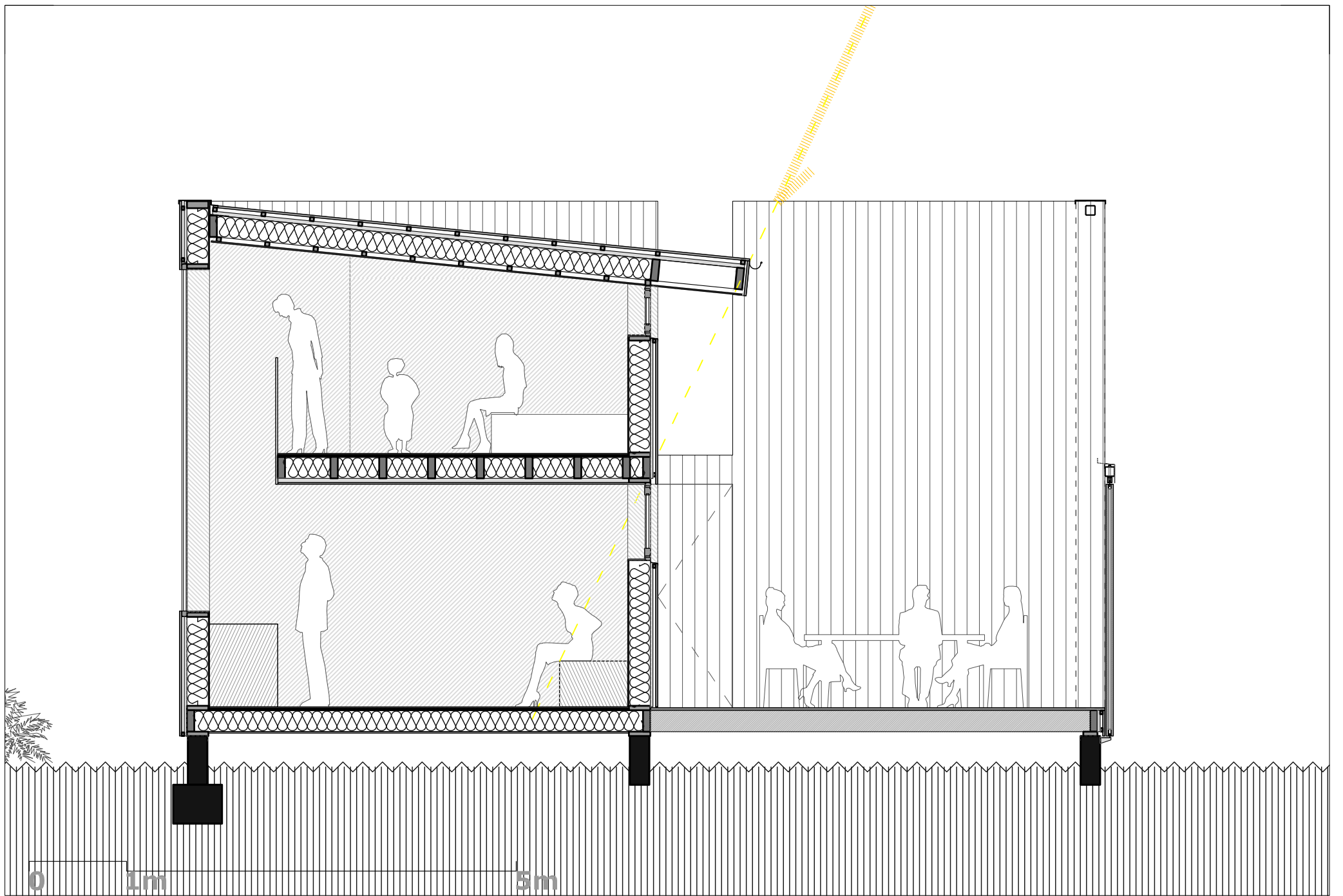
Coupe BB
