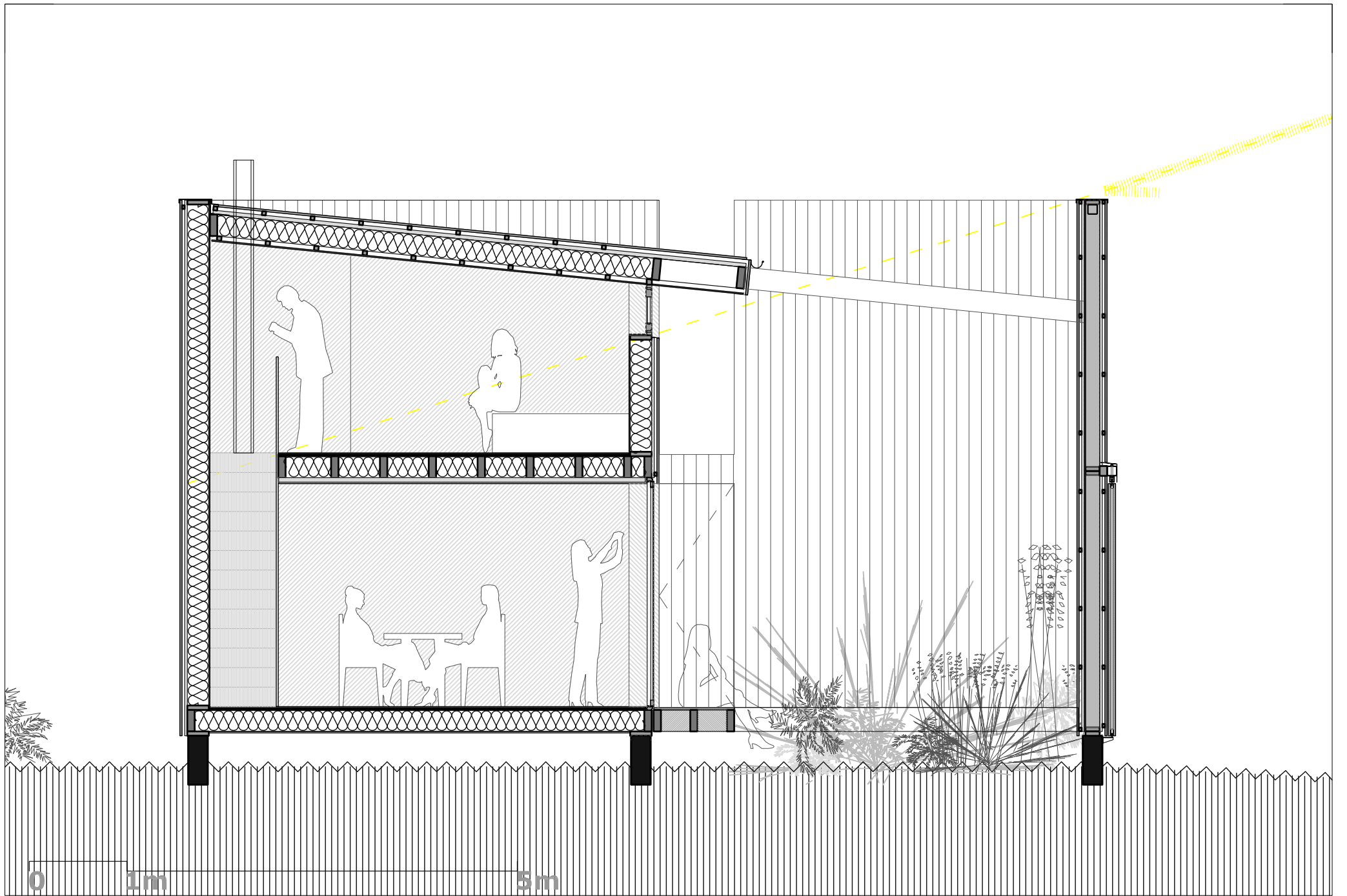
Coupe AA
