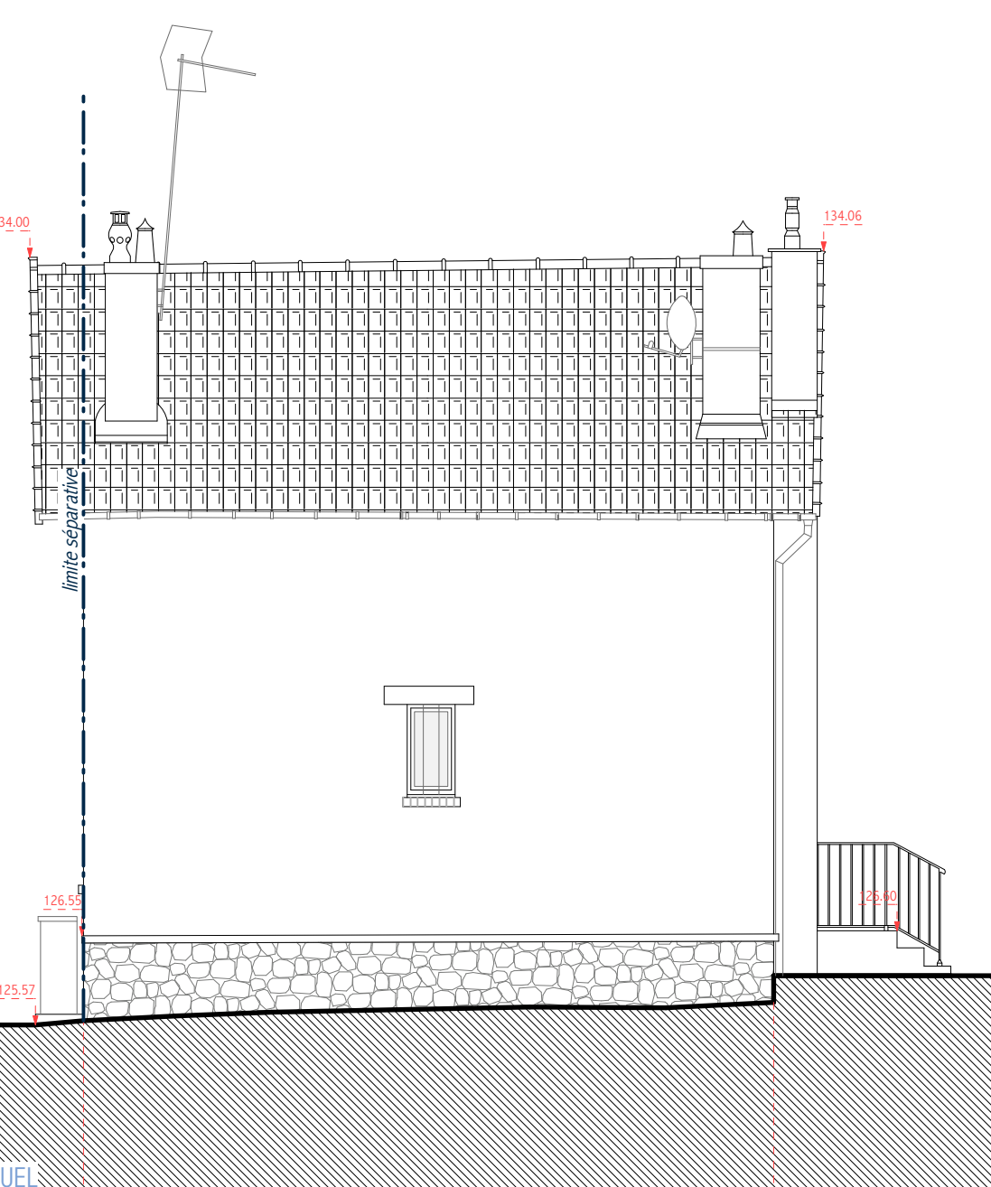
FAÇADE BC - ÉTAT PROJETÉ
