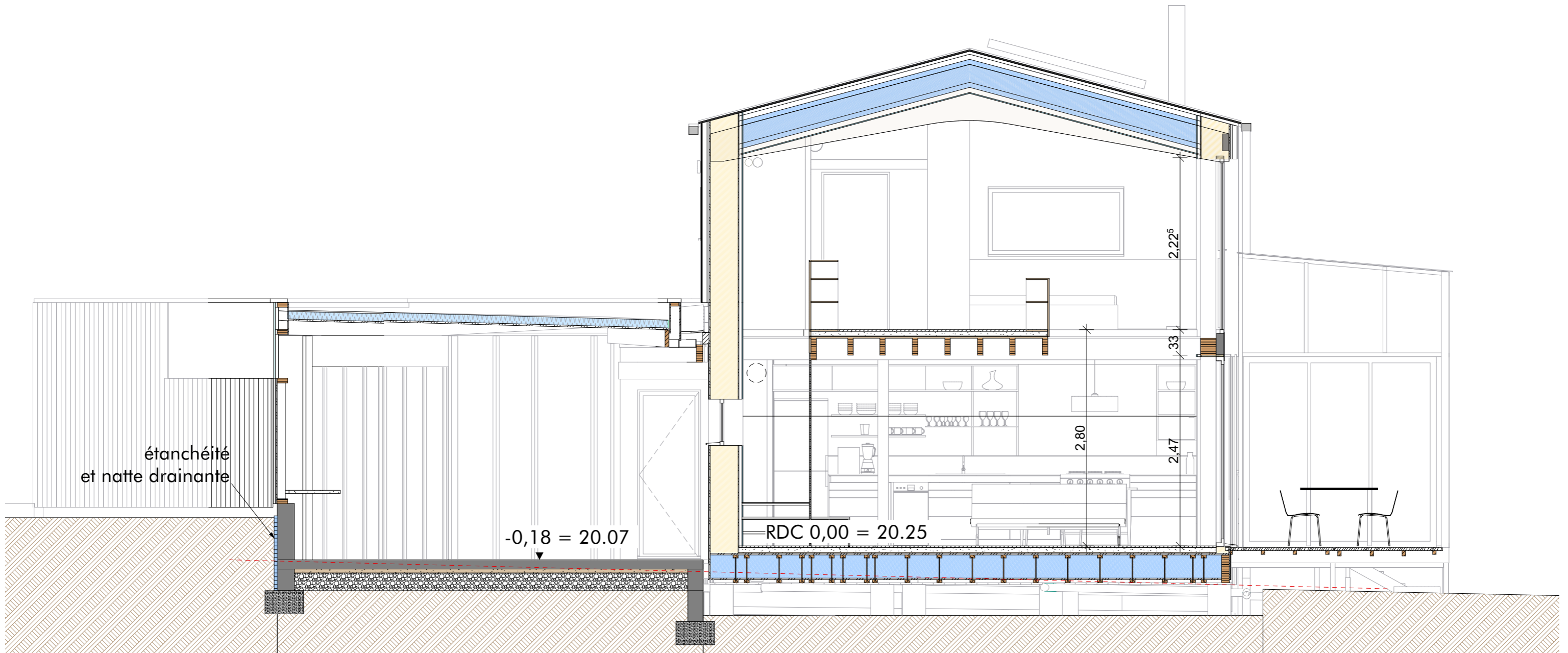
Coupe B4 (1) 1:50
