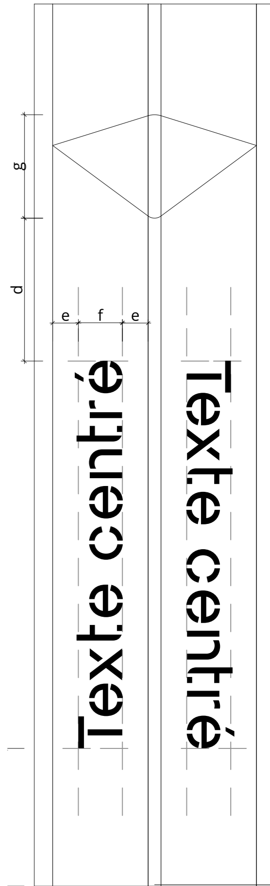
Détail - Positionnement typographie 1:10
