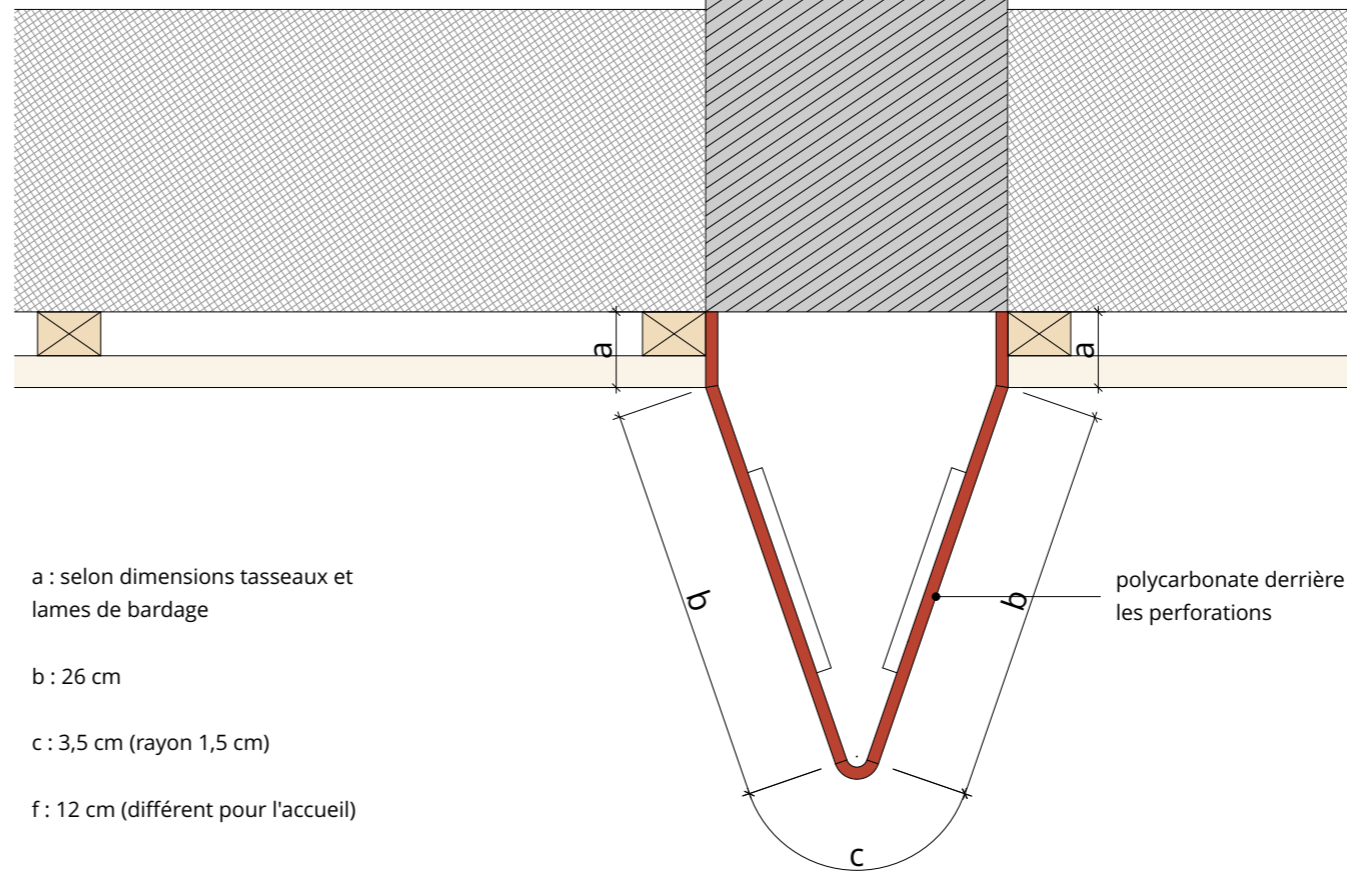
Base nautique de Golfe Juan - Détail plage acier Cor-Ten 1:5
