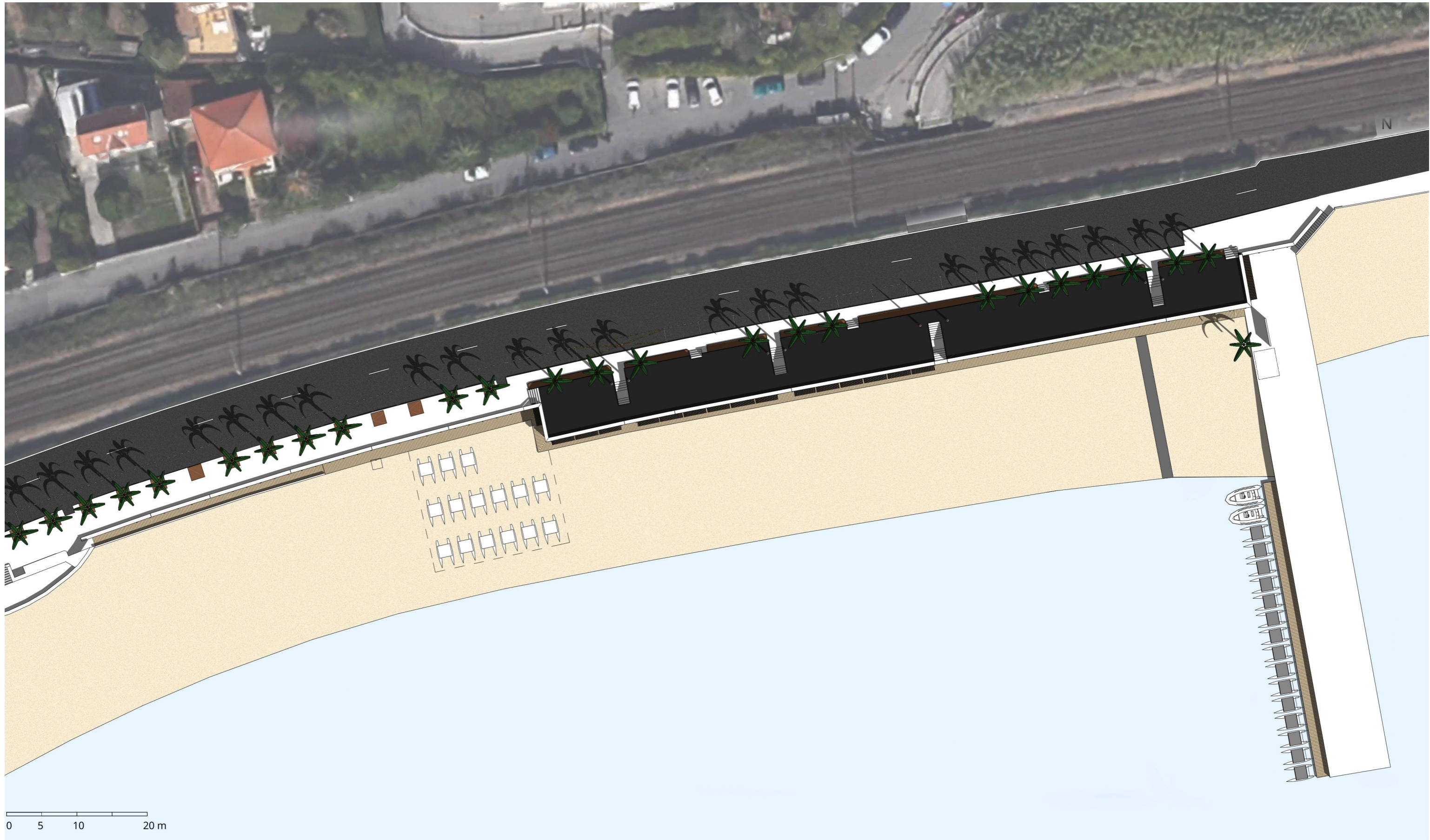
Plan masse 1:500
