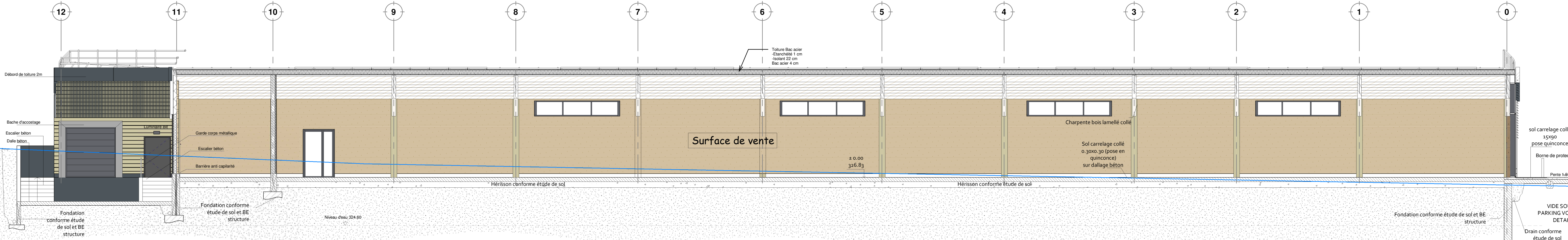
Coupe BB échelle 1 : 100e
