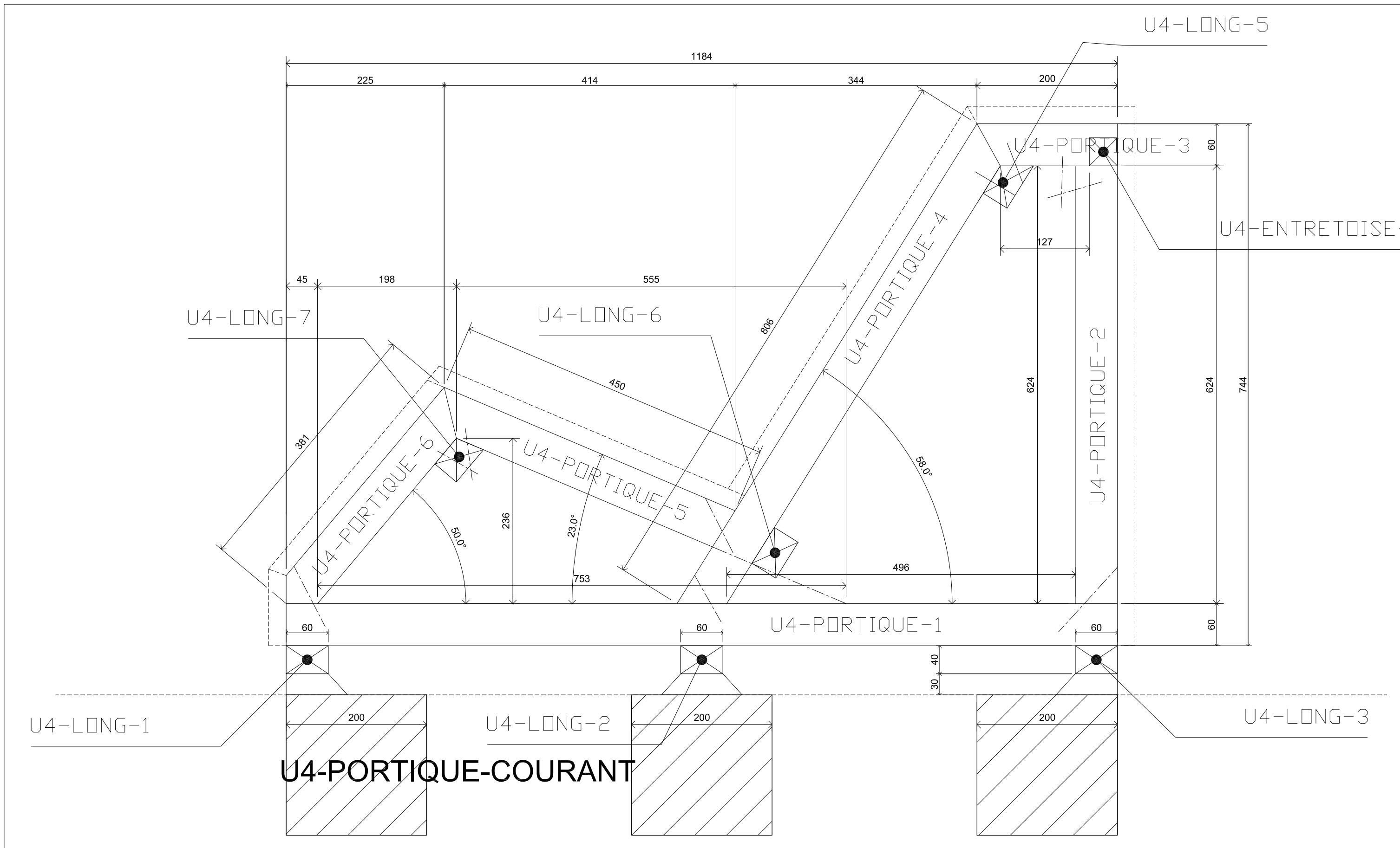
ELEVATION DU PORTIQUE COURANT Nomenclature
